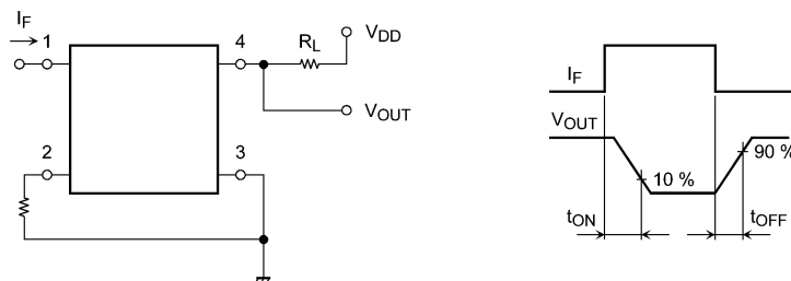
図 11.1 スイッチング時間測定回路, 波形
