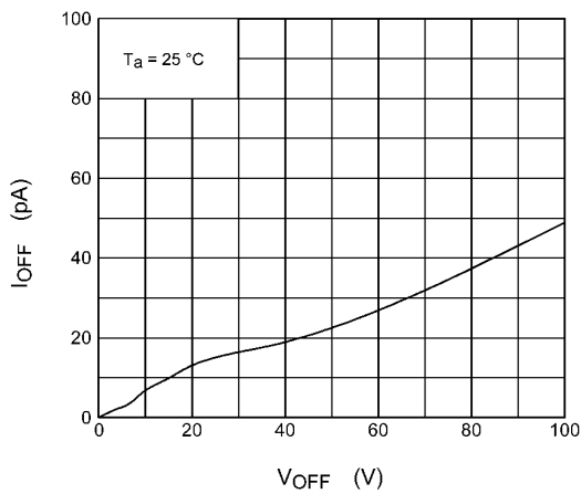
図 12.1.9 I_{OFF} - V_{OFF}
