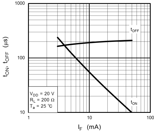
図 12.1.7 t_{ON}, t_{OFF} - I_F
