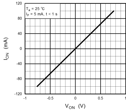
図 12.1.4 I_{ON} - V_{ON}
