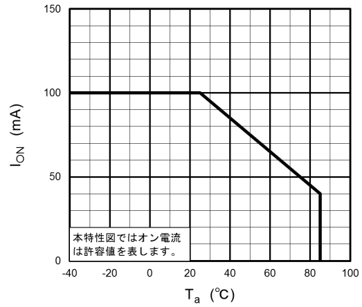
図 12.1.2 I_{ON} - T_a
