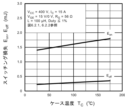
図 8.18 スイッチング損失 - T_C
