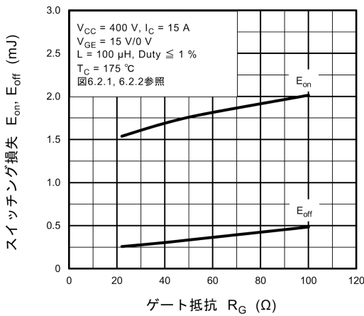
図 8.17 スイッチング損失 - R_G
