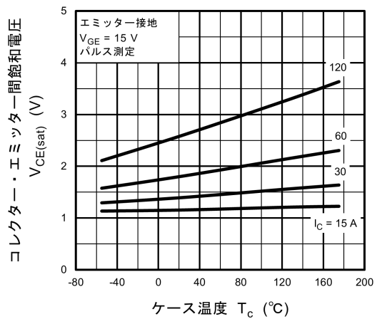
図 8.6 V_{CE(sat)} - T_c
