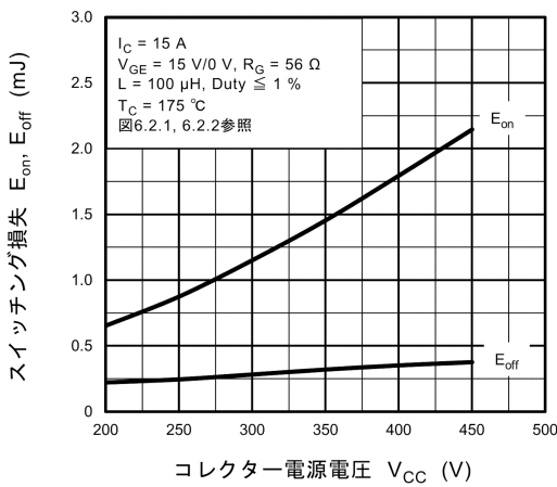
図 8.15 スイッチング損失 - V_{CC}
