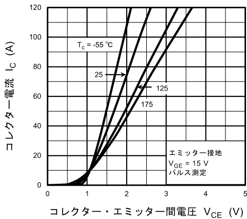
図 8.5 I_C - V_{CE}
