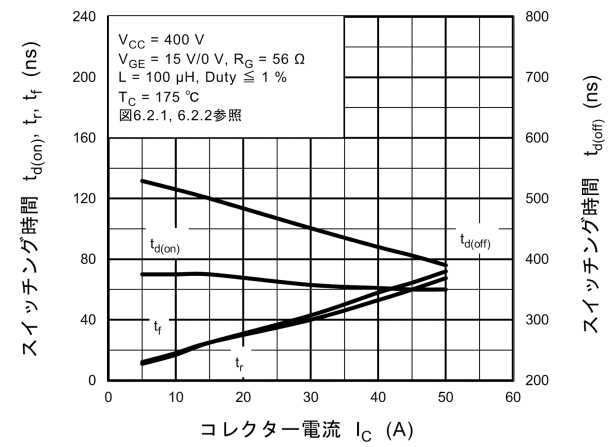
図 8.12 スイッチング時間 - I_C
