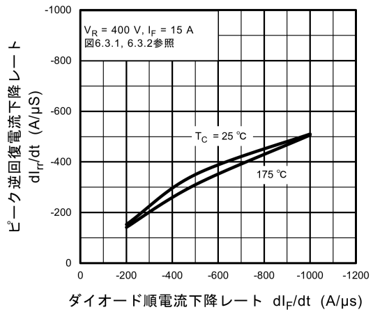
図 8.24 di_{rr}/dt - di_F/dt
