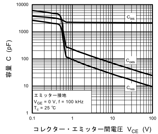
図 8.10 C - V_{CE}
