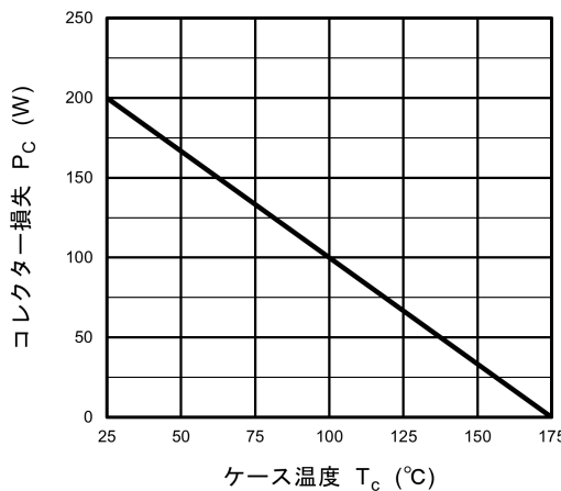
図 8.11 P_C - T_c
