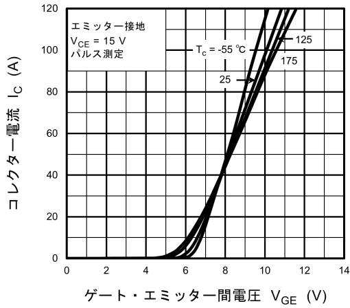
図 8.7 I_C - V_{GE}
