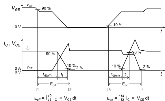
図 6.2.2 タイミングチャート
