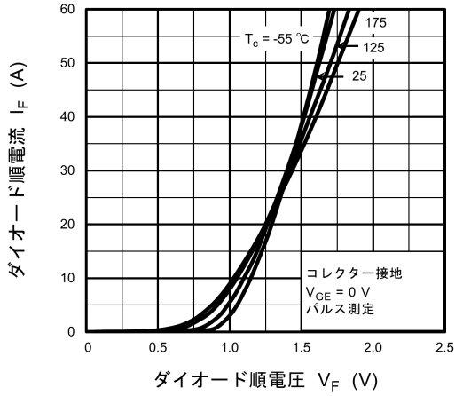
図 8.19 I_F - V_F
