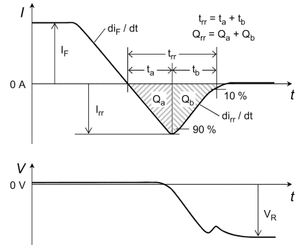
図 6.3.2 タイミングチャート
