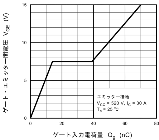
図 8.9 V_{GE} - Q_g
