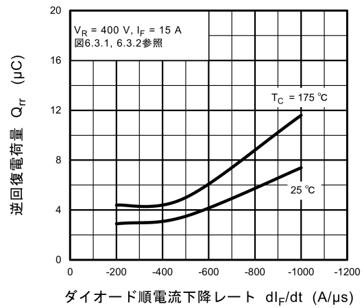
図 8.22 Q_{rr} - di_F/dt
