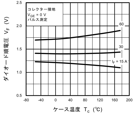
図 8.20 V_F - T_C
