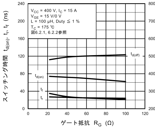
図 8.13 スイッチング時間 - R_G
