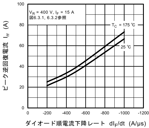
図 8.23 I_{rr} - di_F/dt
