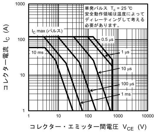
図 8.26 安全動作領域 (最大値 (保証値))
