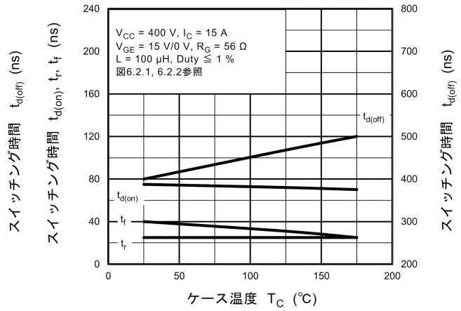
図 8.14 スイッチング時間 - T_C
