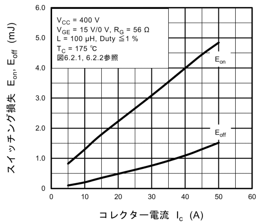
図 8.16 スイッチング損失 - I_C
