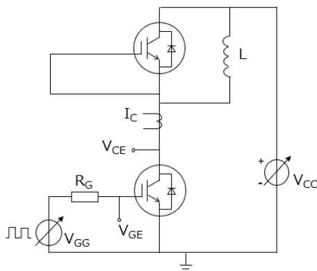
図 6.2.1 測定回路
