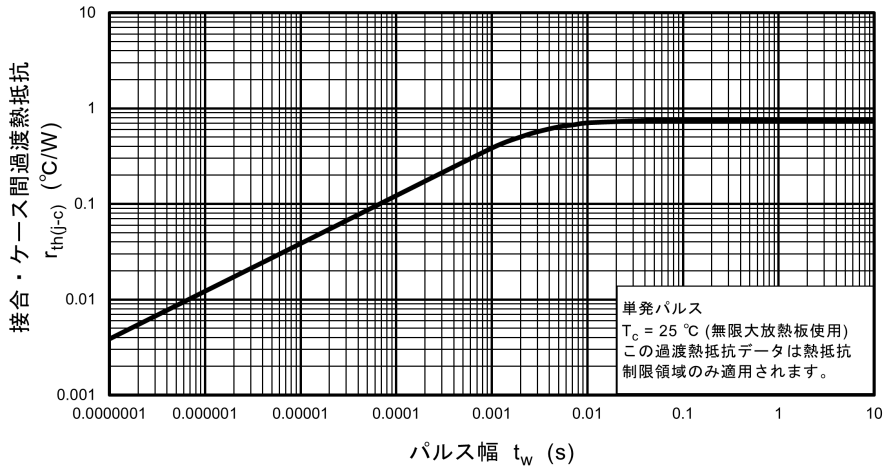
図 8.25 r_{th(j-c)} - t_w (最大値 (保証値))
