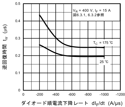
図 8.21 t_{rr} - di_F/dt
