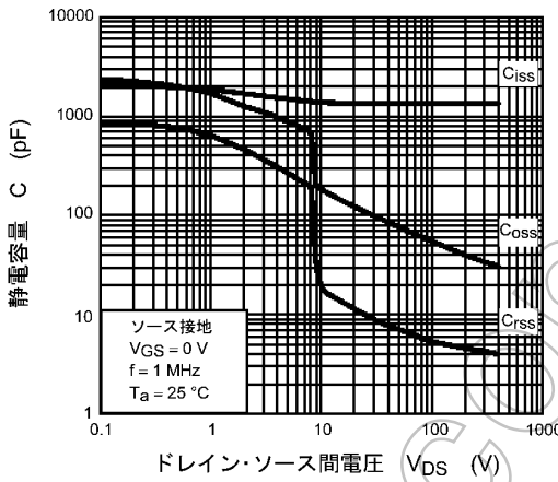
図 8.9 C - V_{DS}
