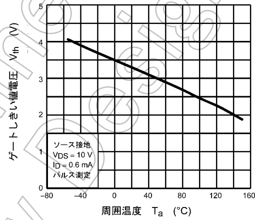
図 8.10 V_{th} - T_a
