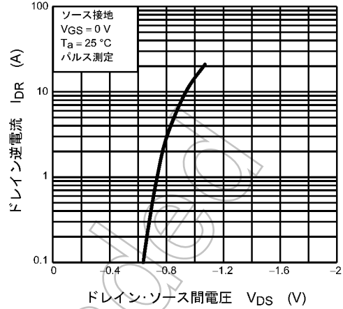
図 8.8 I DR - V DS
