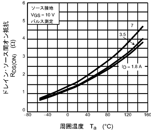
図 8.7 R DS(ON) - T a
