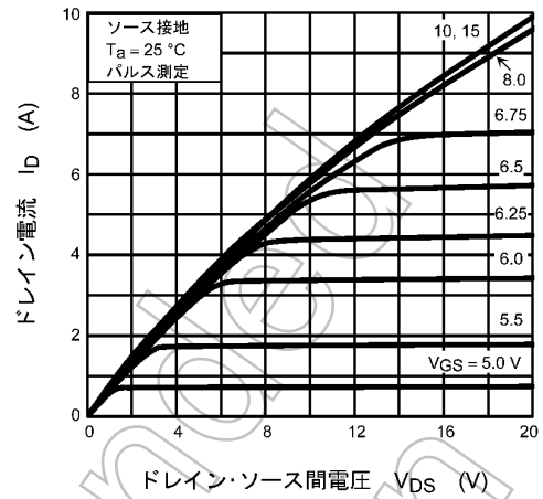
図 8.2 I_D - V_{DS}
