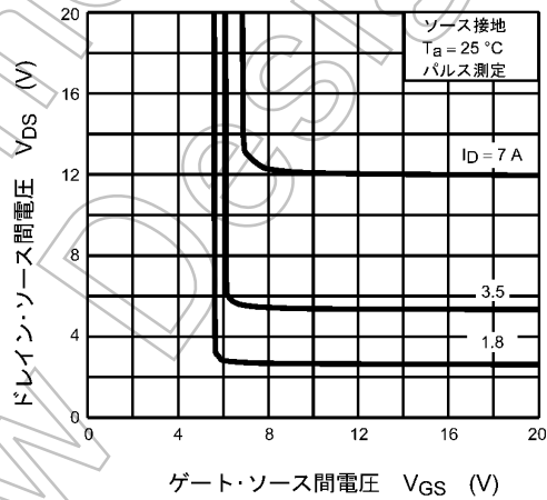
図 8.4 V_{DS} - V_{GS}
