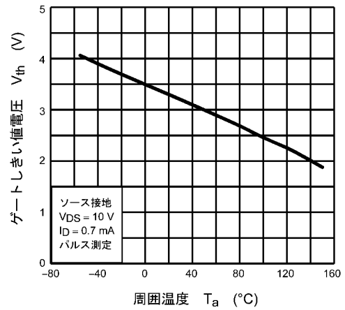
図 8.10 V_{th} - T_a
