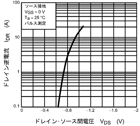
図 8.8 I_{DR} - V_{DS}
