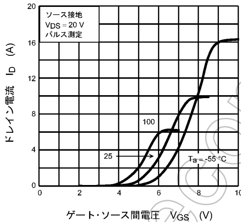
図 8.3 I_D - V_{GS}
