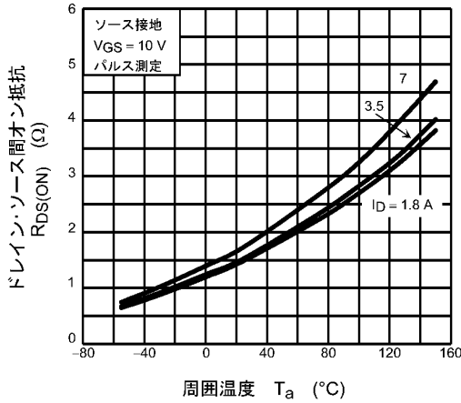
図 8.7 R_{DS(ON)} - T_a
