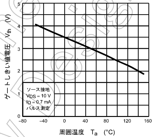
図 8.10 V_{th} - T_a
