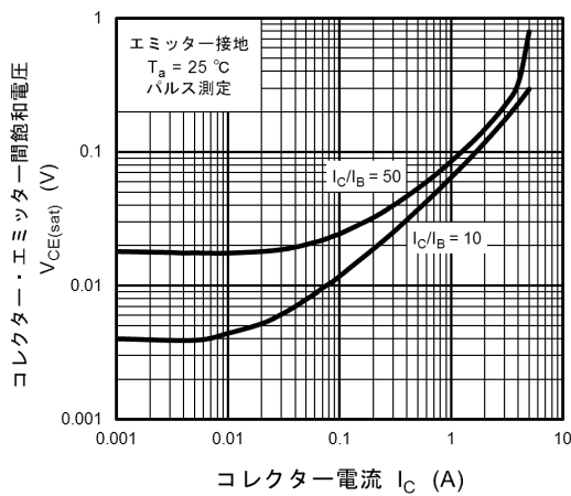
図 7.5 V_{CE(sat)} - I_C
