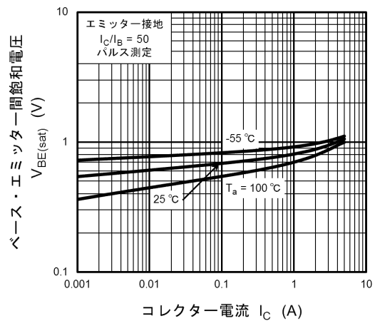
図 7.6 V_{BE(sat)} - I_C
