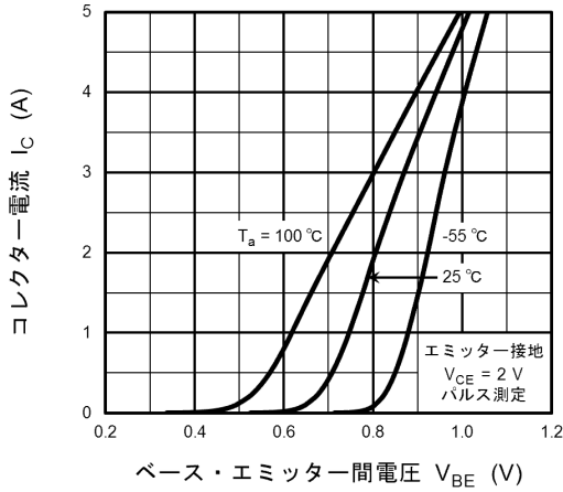
図 7.7 IC - V BE
