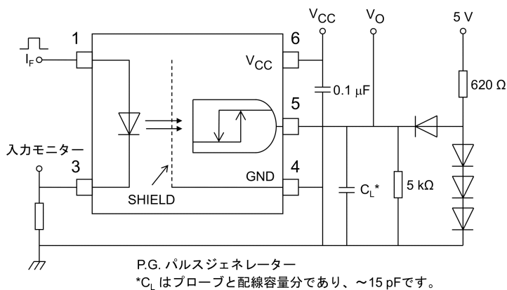
図 12.1.7 伝搬遅延時間測定回路, 波形
