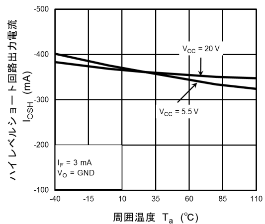
図 12.2.10 I_{osH} - T_a
