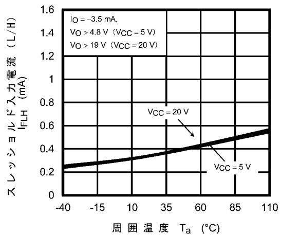
図 12.2.2 I_{FLH} - T_a
