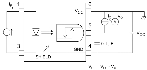
図 12.1.2 V_{OH} 測定回路
