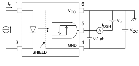
図 12.1.6 I_{OSH} 測定回路
