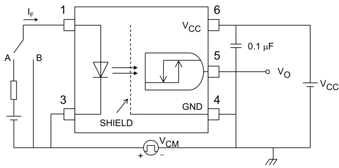
図 12.1.9 コモンモード過渡耐性測定回路, 波形
