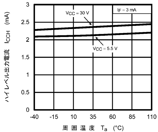
図 12.2.8 I_{cCH} - T_a
