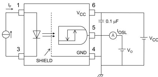
図 12.1.5 I_{OSL} 測定回路
