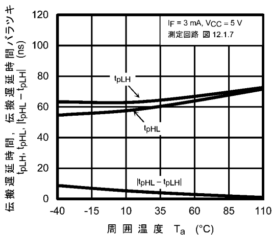
図 12.2.11 t_{pLH}, t_{pHL}, |t_{pHL} - t_{pLH}| - T_a (測定回路 図12.1.7)
