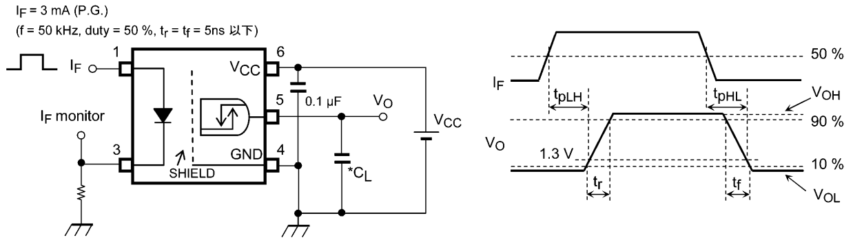
図 12.1.8 伝搬遅延時間測定回路, 波形
