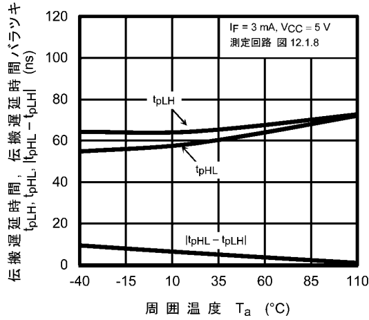
図 12.2.13 t_{pLH} , t_{pHL} , |t_{pHL} - t_{pLH}| - T_a (測定回路 図12.1.8)
