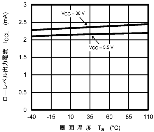
図 12.2.7 I_{cCL} - T_a
