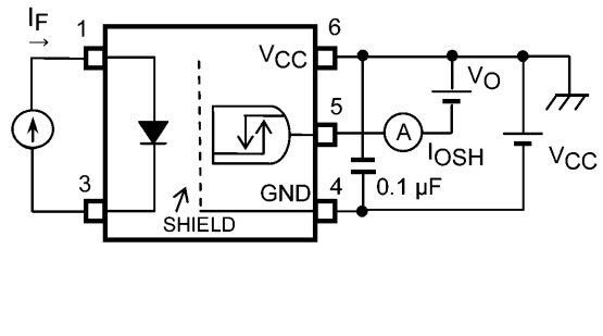
図 12.1.6 IOSH測定回路
