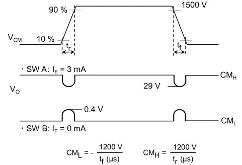
図 12.1.9 コモンモード過渡耐性測定回路, 波形
