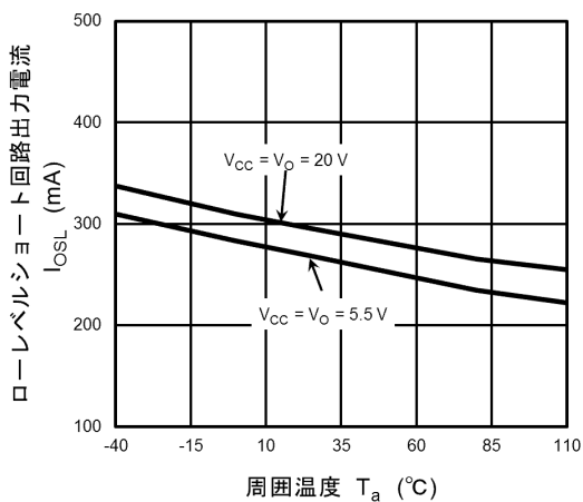
図 12.2.9 I_{osL} - T_a
