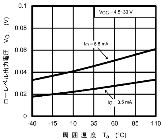
図 12.2.5 V_{OL} - T_a
