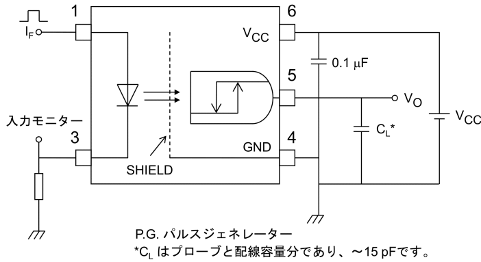
図 12.1.8 伝搬遅延時間測定回路, 波形
