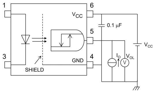
図 12.1.1 V_{OL} 測定回路
