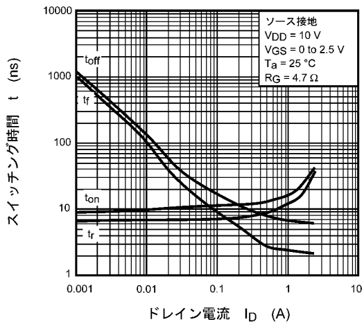
図 7.1.11 t - I_D
