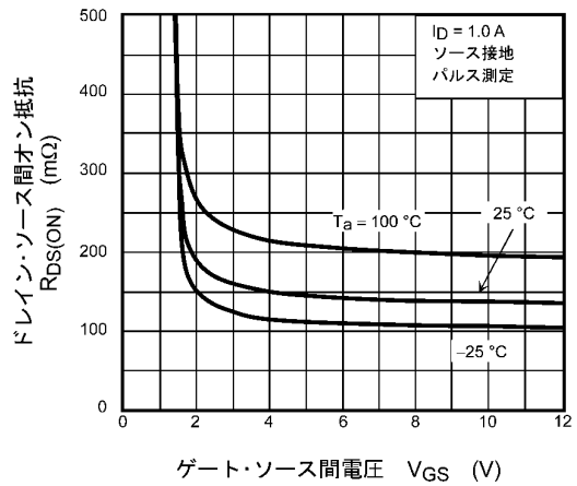
図 7.1.4 R_{DS(ON)} - V_{GS}
