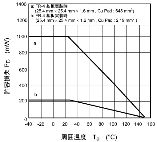
図 7.3.2 P_D - T_a
