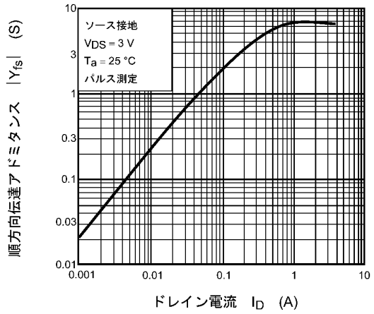
図 7.1.8 |Y_{fs}| - I_D
