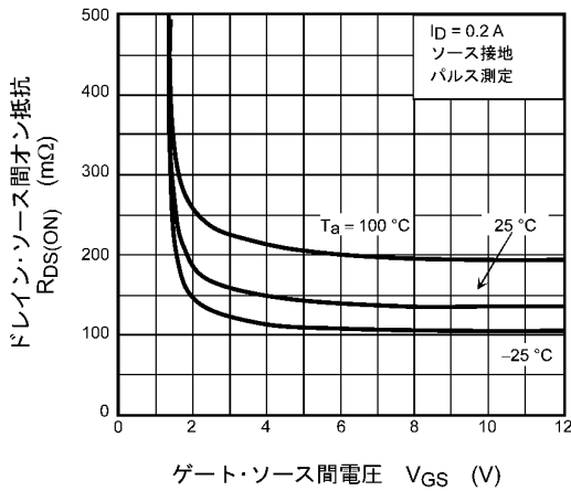
図 7.1.3 R_{DS(ON)} - V_{GS}
