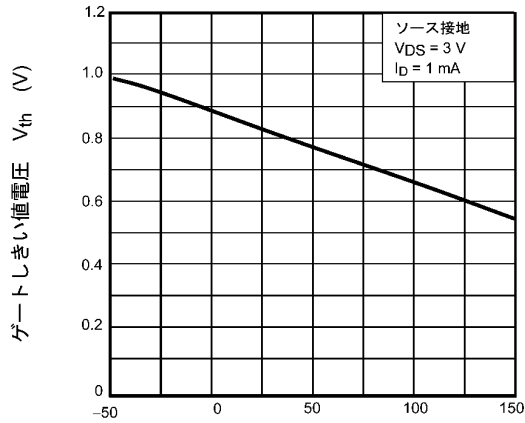
図 7.1.7 V_{th} - T_a
