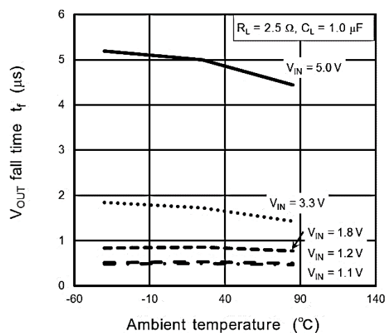
t_f - T_a
