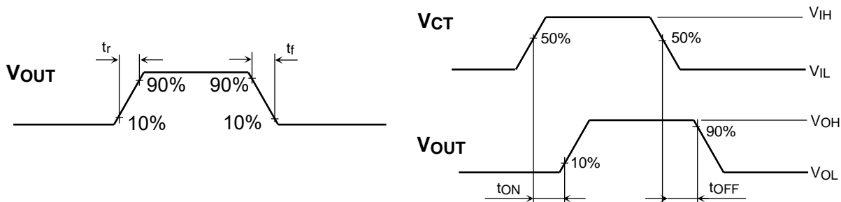
図 1: t r , t f , t ON , t OFF 波形
