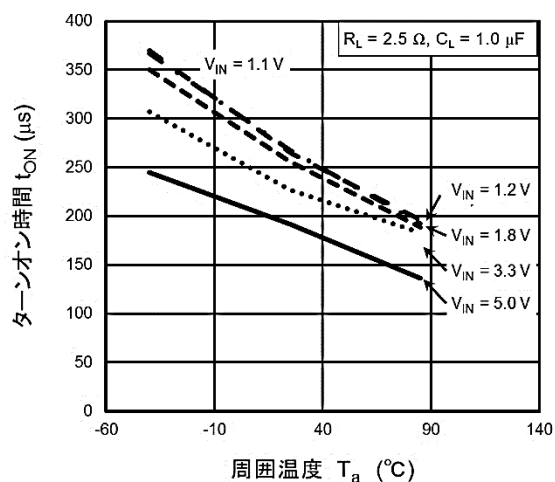
t_{ON} - T_a
