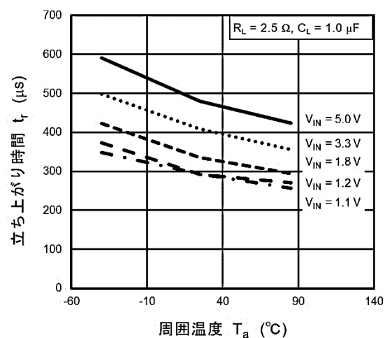
t_r - T_a
