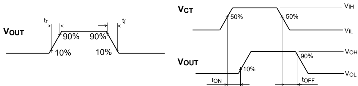
図 1: t r , t f , t ON , t OFF 波形
