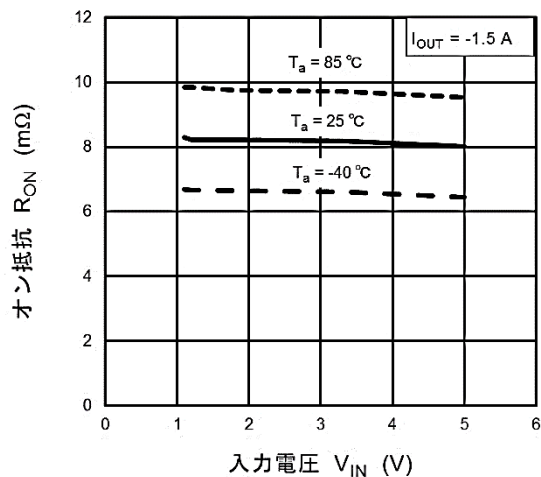
R_{ON} - V_{IN}
