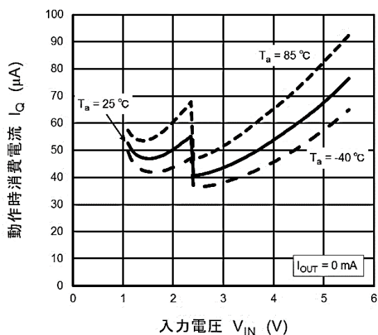
I_Q - V_{IN}
