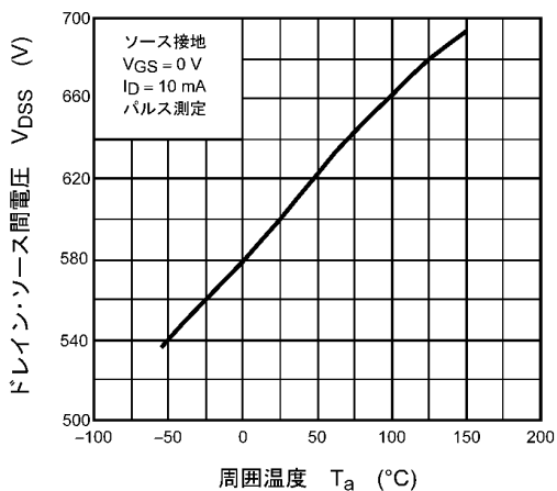
図 8.5 V_{DSS} - T_a
