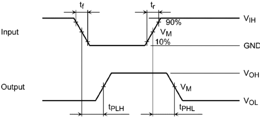
図 9.7.1 t_{PLH} , t_{PHL}
