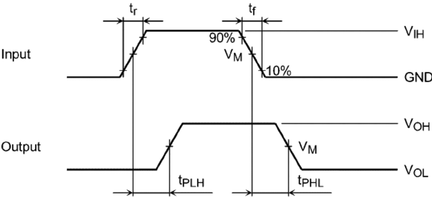
図 9.7.1 t_{PLH}, t_{PHL}
