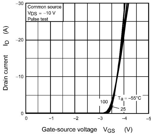
Fig. 8.3 I_D - V_{GS}
