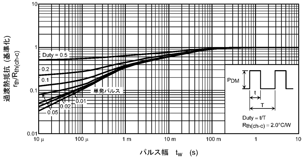
図 8.11 r_{th} - t_w (最大値 (保証値))
