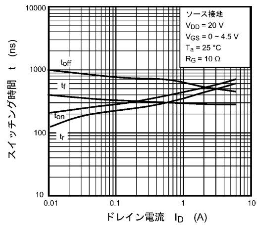
図 7.10 t - I_D
