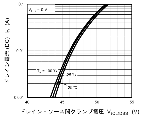
図 7.12 I_D - V_{(CL)DSS}
