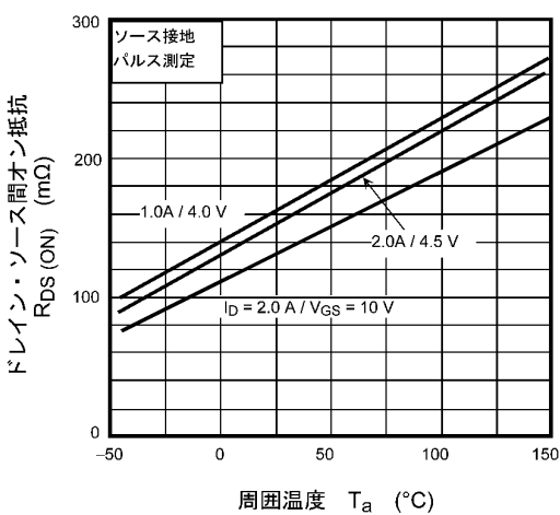
図 7.5 R_{DS(ON)} - T_a
