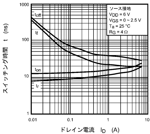
図 7.11 t - I_D
