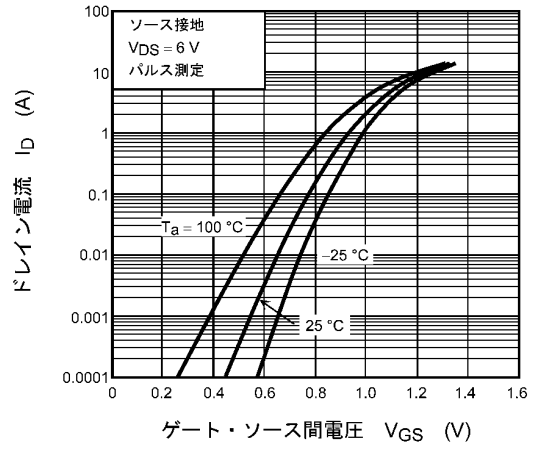
図 7.2 I_D - V_{GS}
