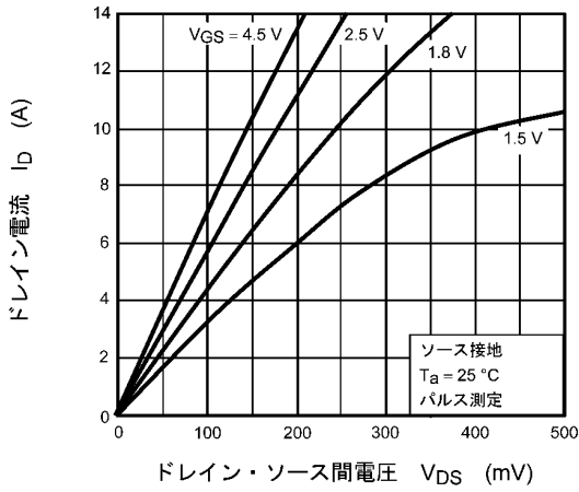
図 7.1 I_D - V_{DS}
