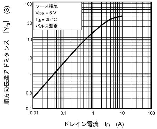
図 7.8 |Y_{fs}| - I_D
