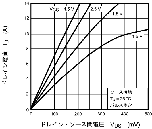
図 7.1 I_D - V_{DS}
