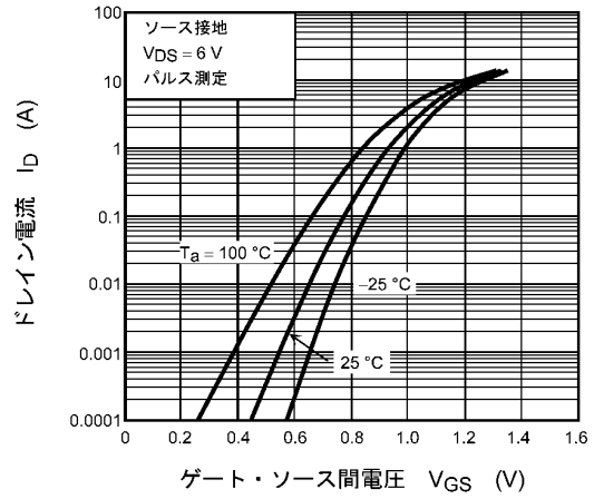
図 7.2 I_D - V_{GS}
