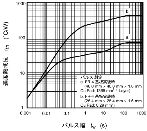
図 7.13 r_{th} - t_w
