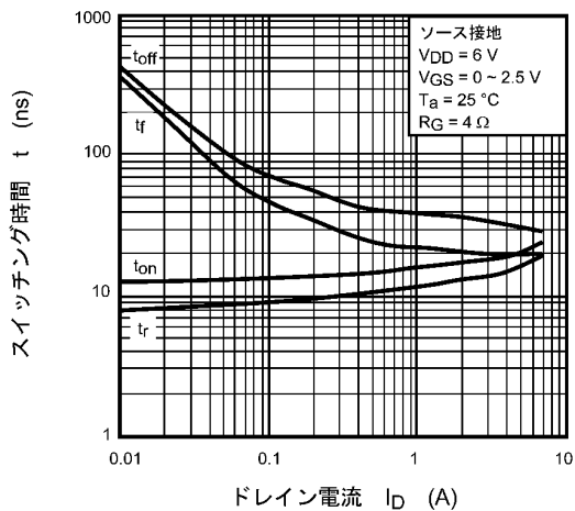
図 7.11 t - I_D
