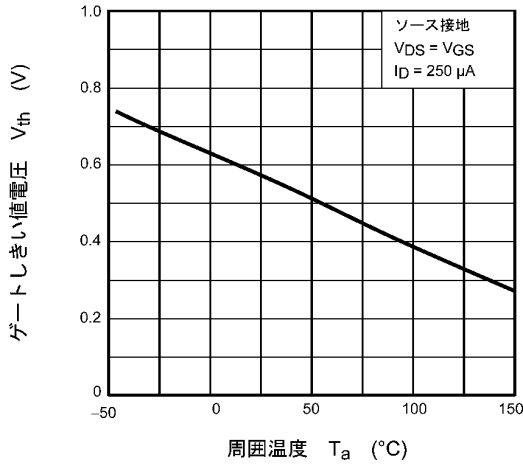
図 7.7 V_{th} - T_a
