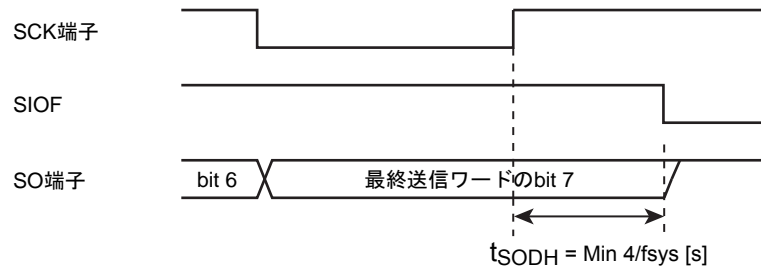
14-21 送信終了時の最終ビット保持時間
