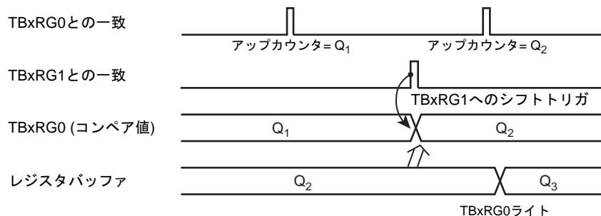
図 11-3 レジスタバッファの動作
