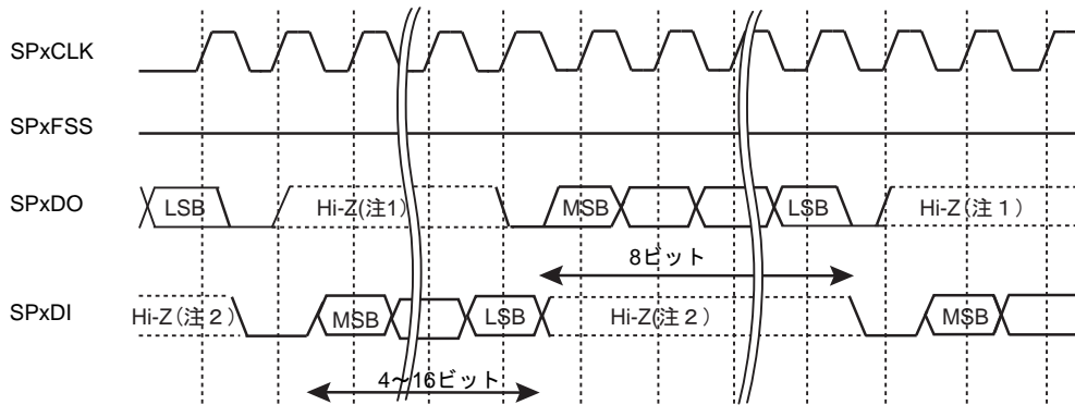
図 15-11 Microwire フレームフォーマット（連続転送）
