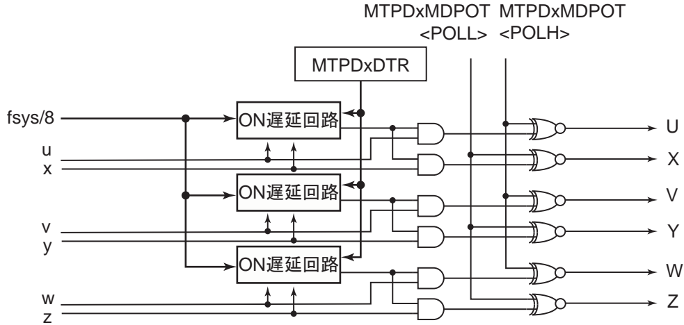
図 18-28 デッドタイム回路概略図
