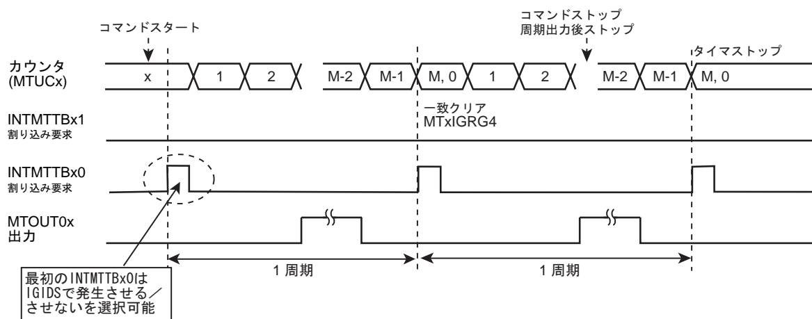
図 18-7 周期割り込み動作
