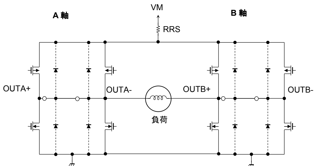
図 7.2 1 DC motor (Large mode) 組み合わせの接続図
