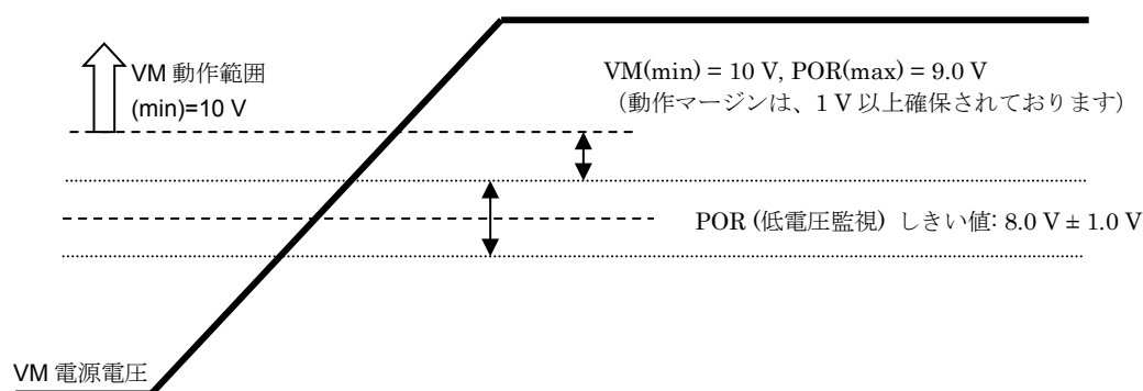
図 1.1 電源電圧と動作範囲
