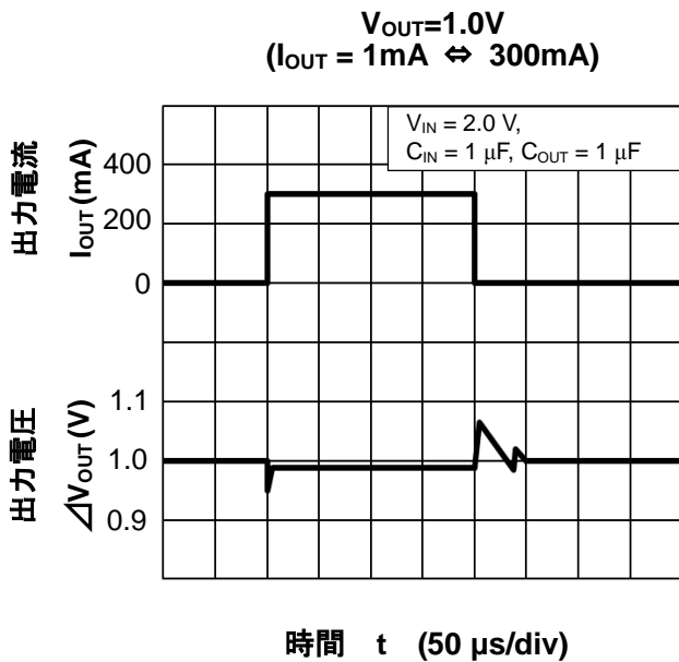
負荷過渡応答特性
