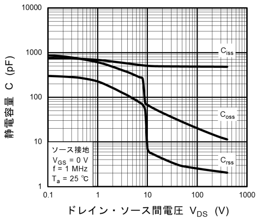
図 8.9 C - V_{DS}
