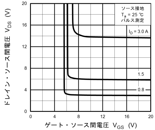
図 8.4 V_{DS} - V_{GS}
