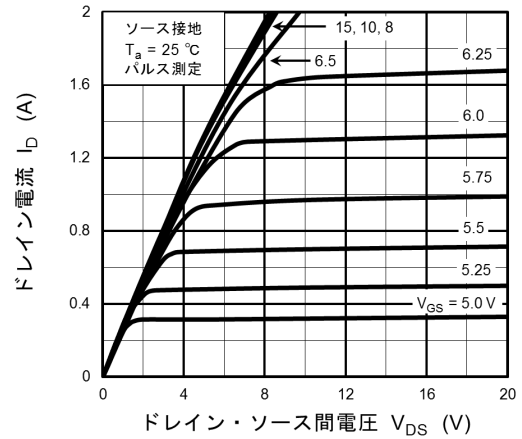
図 8.2 I_D - V_{DS}
