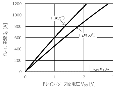
図 4.4.1 I_D - V_{DS(on)sense} 特性の例
