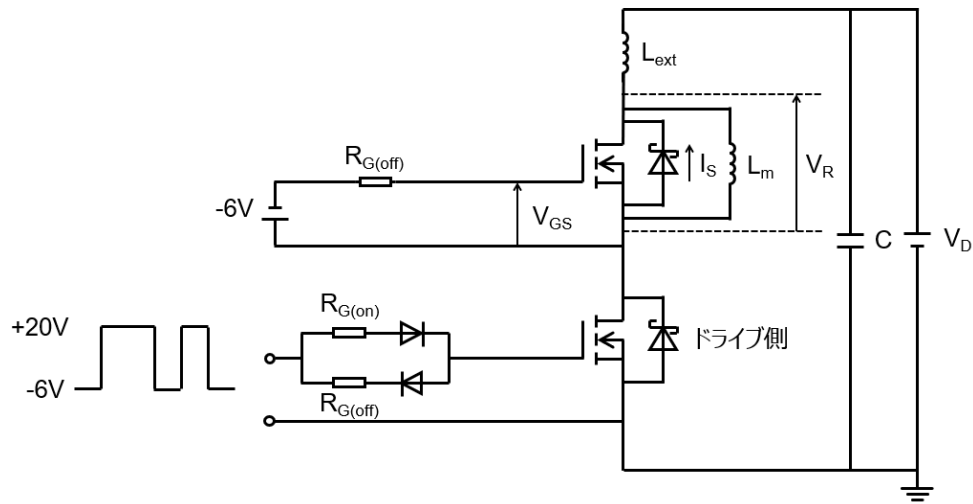
a) 逆回復測定回路（誘導負荷、ローサイド逆回復の例）
