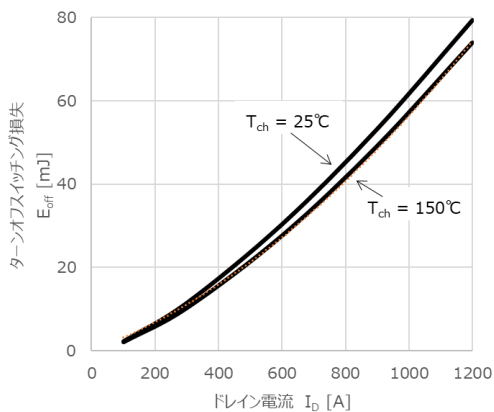
図 5.8.2 E_{off} - I_D 特性の例
