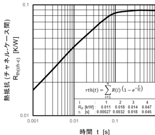
図 3.1.2 r_{th(ch-c)} - t 特性の例
