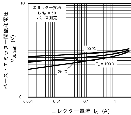
図 7.4 V_{BE(sat)} - I_C
