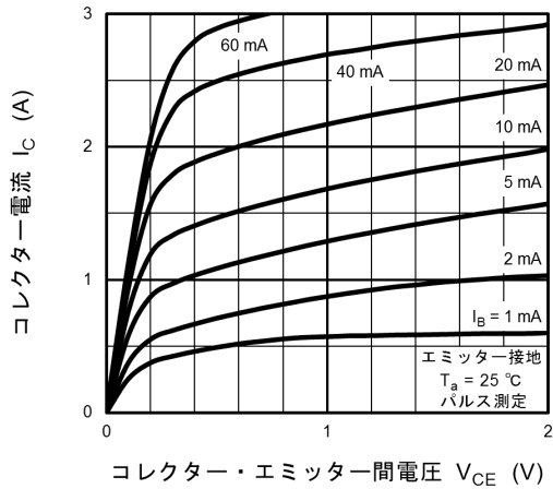
図 7.1 I_C - V_{CE}
