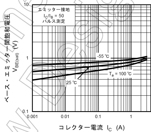
図 7.4 V_{BE(sat)} - I_C
