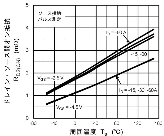
図 8.6 R_{DS(ON)} - T_a
