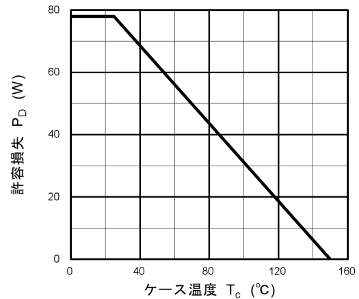
図 8.12 P_D - T_c (最大値 (保証値))
