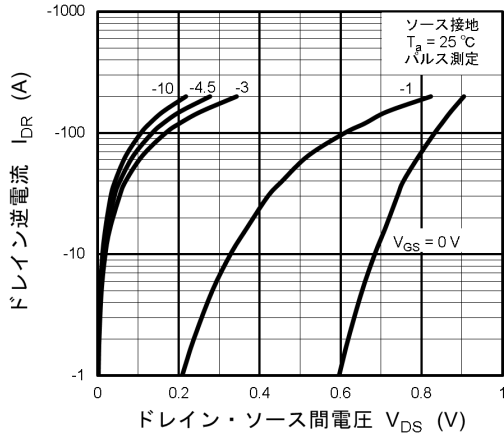
図 8.7 I_{DR} - V_{DS}
