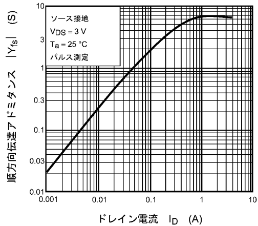
図 8.8 |Y_{fs}| - I_D
