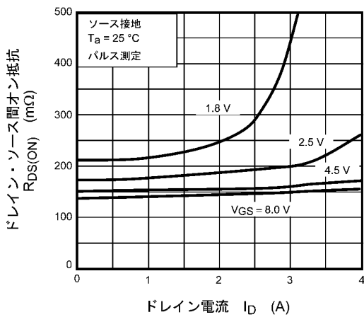
図 8.5 R_{DS(ON)} - I_D
