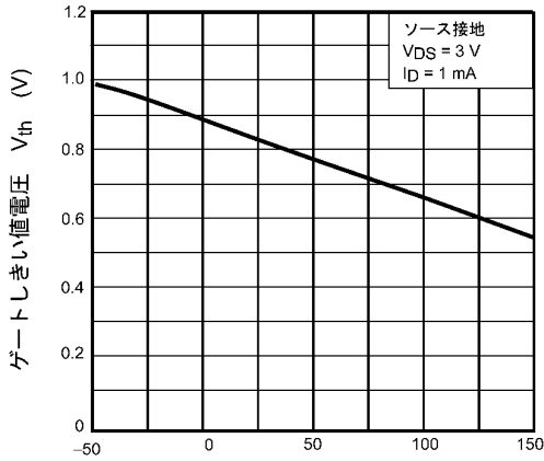
図 7.7 V_{th} - T_a
