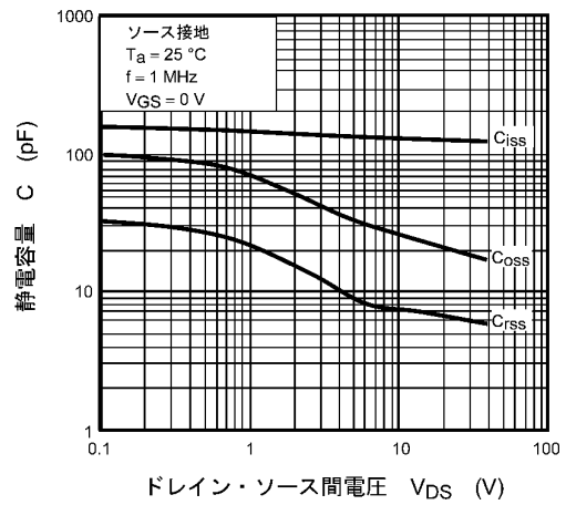
図 7.10 C - V_{DS}
