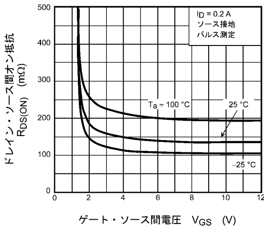
図 8.3 R_{DS(ON)} - V_{GS}
