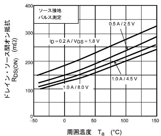
図 7.6 R_{DS(ON)} - T_a
