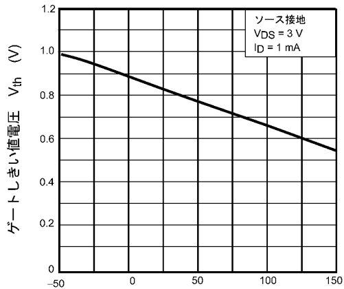
図 8.7 V_{th} - T_a
