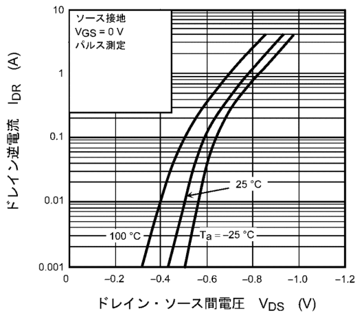
図 8.9 I_{DR} - V_{DS}
