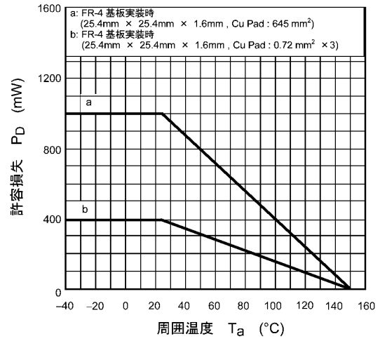
図 8.14 P_D - T_a
