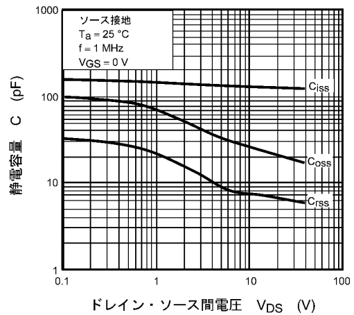
図 8.10 C - V_{DS}
