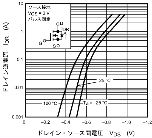
図 7.9 I_{DR} - V_{DS}
