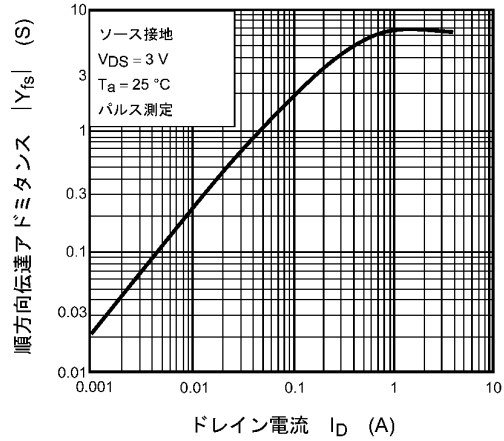
図 7.8 |Y_{fs}| - I_D
