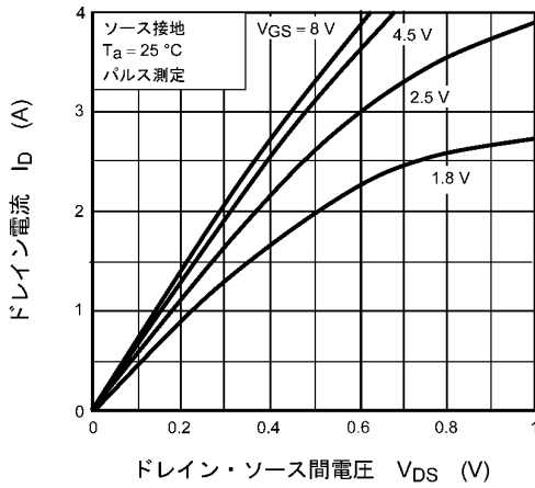
図 7.1 I_D - V_{DS}
