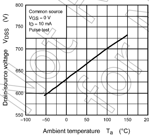
Fig. 8.5 V_{DS} - T_a
