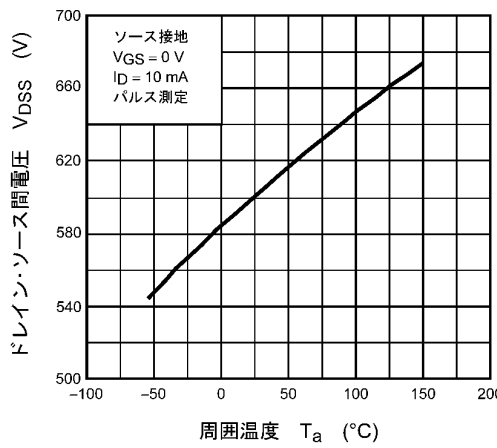
図 8.5 V_{DS} - T_a
