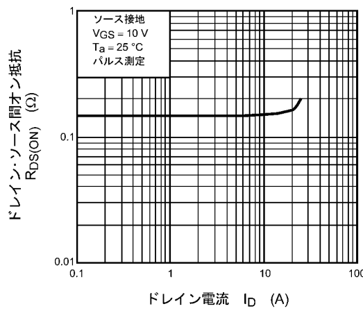
図 8.6 R_{DS(ON)} - I_D
