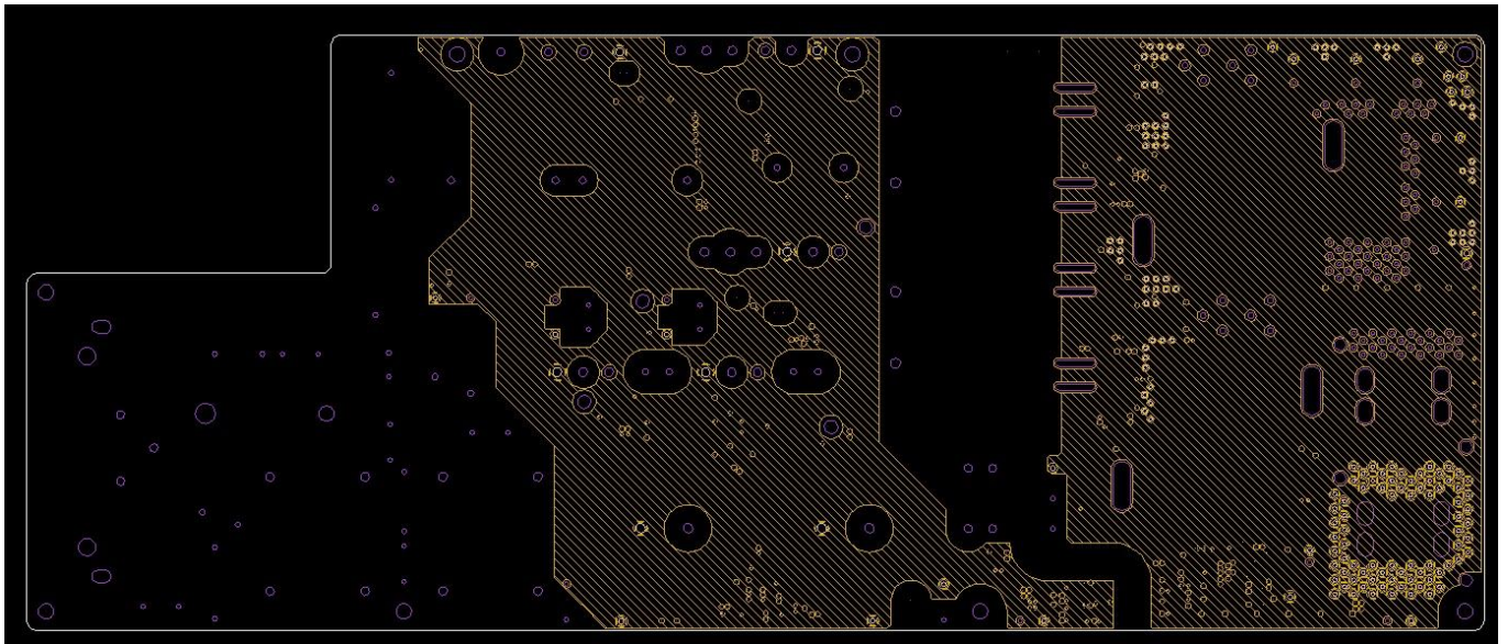
図 2.5.2 Layer2
