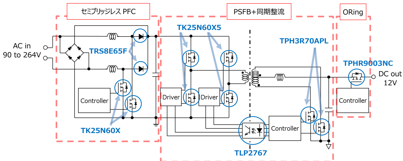
図 2.3.1 ブロック図
