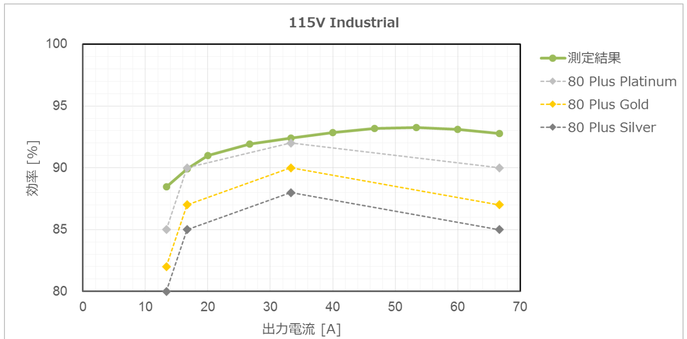
図 4.1.3 効率測定結果(80 PLUS:115V Industrial)
