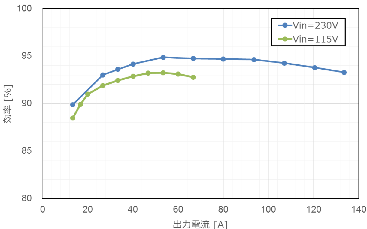
図 4.1.1 効率測定結果(VinAC=115V, VinAC=230V)
