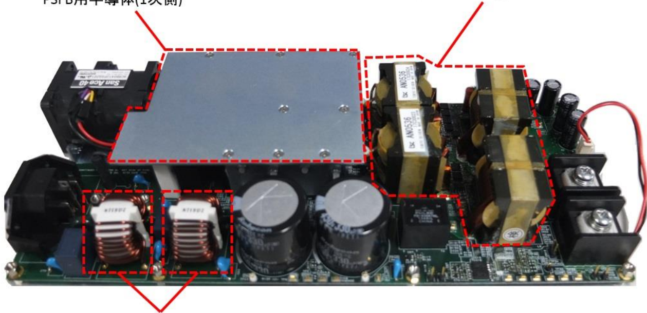
図 3.3.2 発熱量の大きな部品領域
