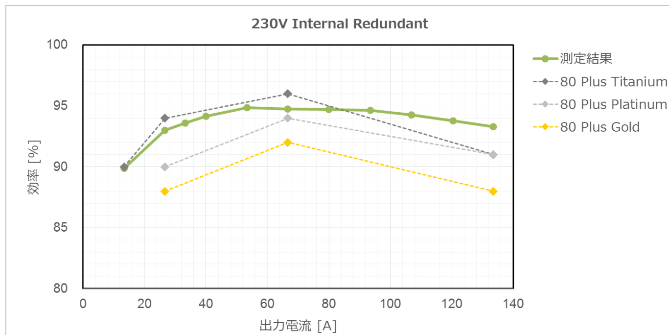
図 4.1.5 効率測定結果(80 PLUS:230V Internal Redundant)
