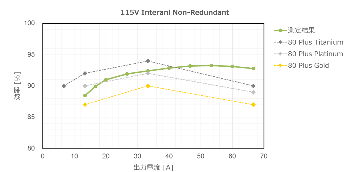
図 4.1.2 効率測定結果(80 PLUS:115V Internal Non-Redundant)
