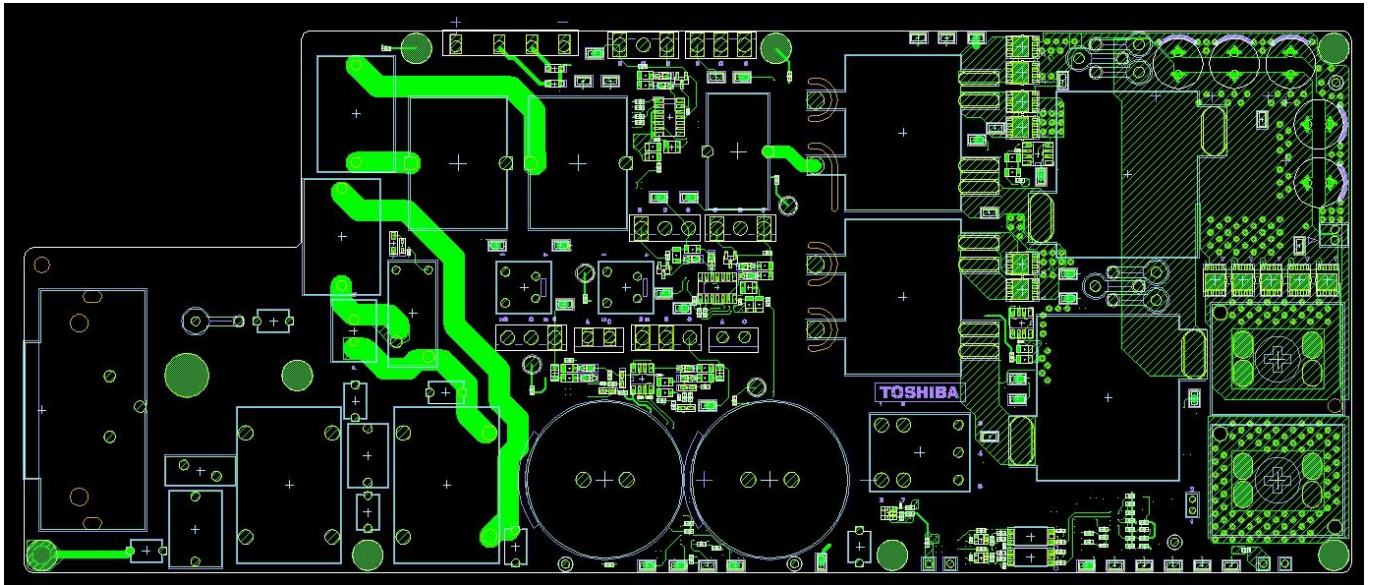
図 2.5.1 Layer1
