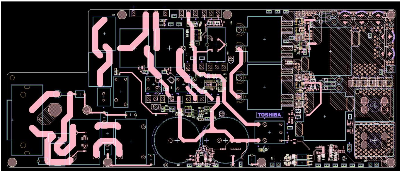
図 2.5.6 Layer6
