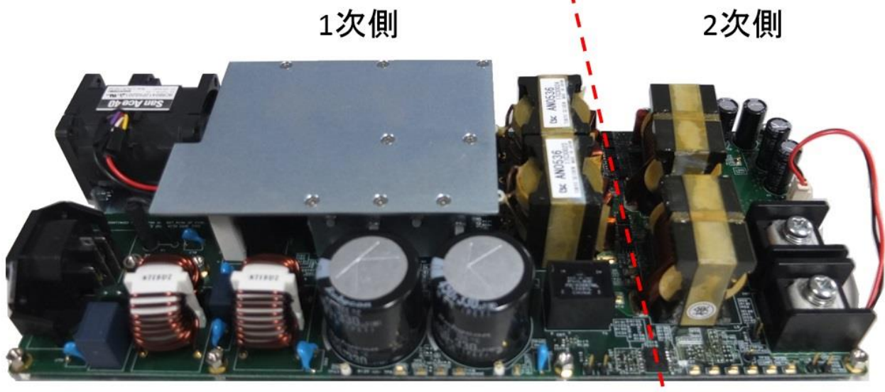
図 3.3.1 1 次側領域と 2 次側領域
