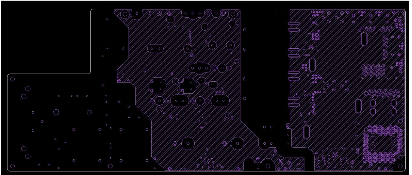
図 2.5.5 Layer5
