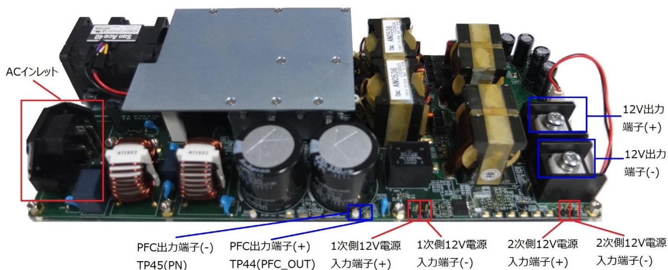
図 3.1.1 外部接続端子
