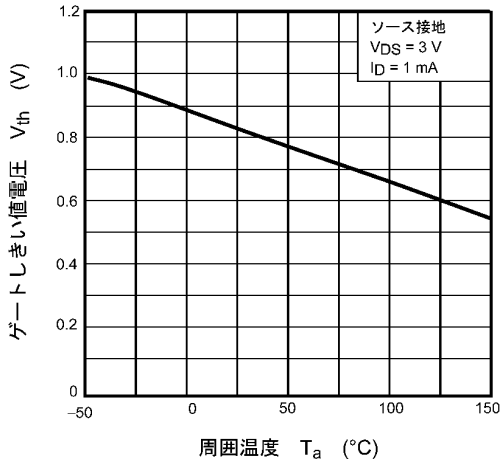
図 7.7 V_{th} - T_a
