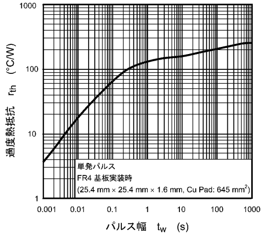
図 7.13 r_{th} - t_w
