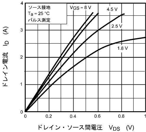
図 7.1 I_D - V_{DS}
