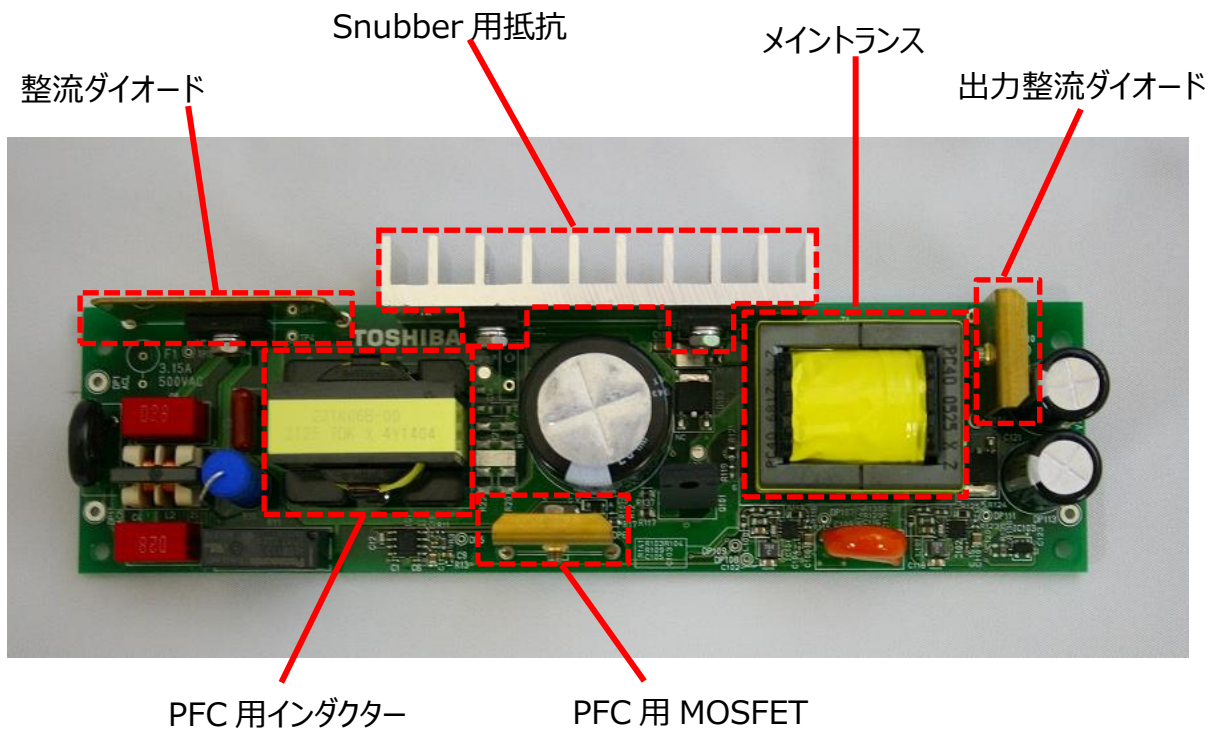
図 3.3 発熱量の大きな部品領域
