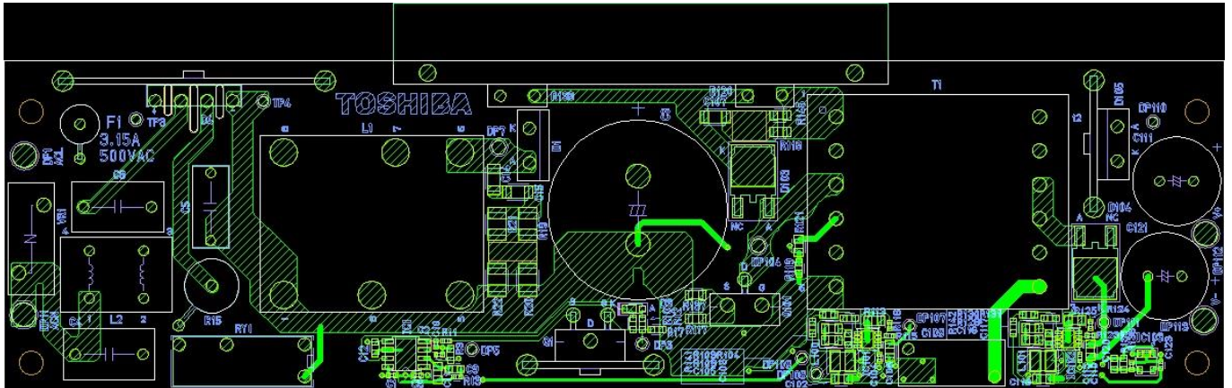
図 2.5 Layer1
