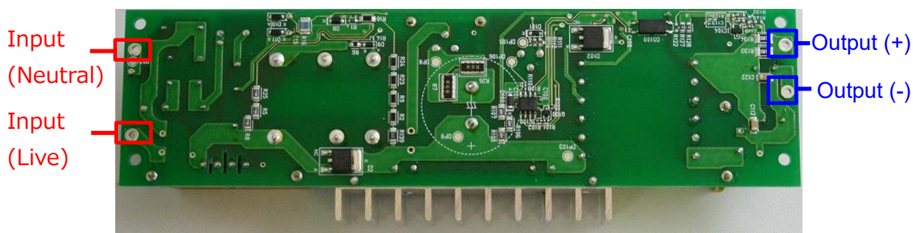
図 3.1 外部接続端子
