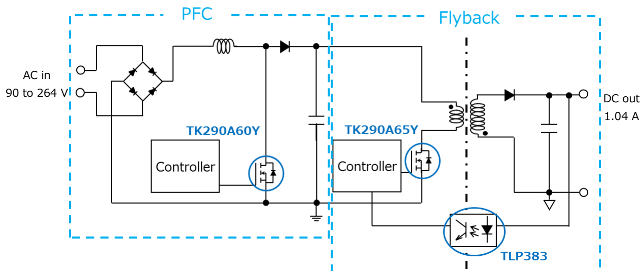
図 2.2 ブロック図
