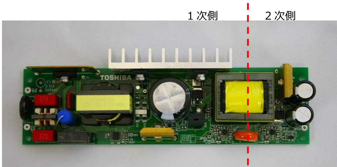
図 3.2 1 次側領域と 2 次側領域
