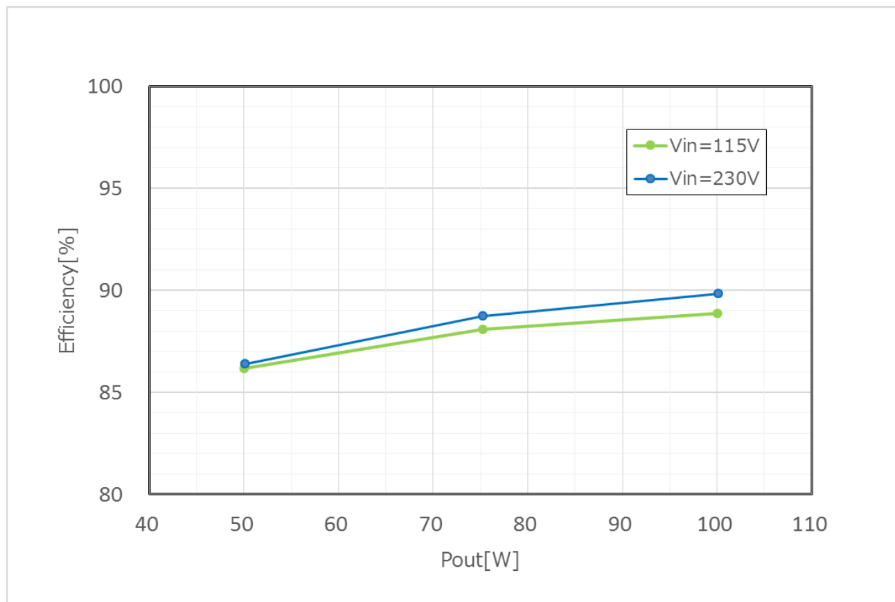
図 4.1 効率測定結果 ( I_{out} = 1.04 \text{ A} , V_{inAC} = 115 \text{ V} , V_{inAC} = 230 \text{ V} )
