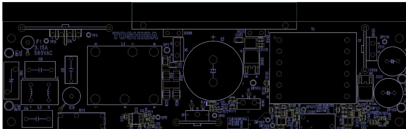
図 2.3 PCB 部品配置 (表面)
