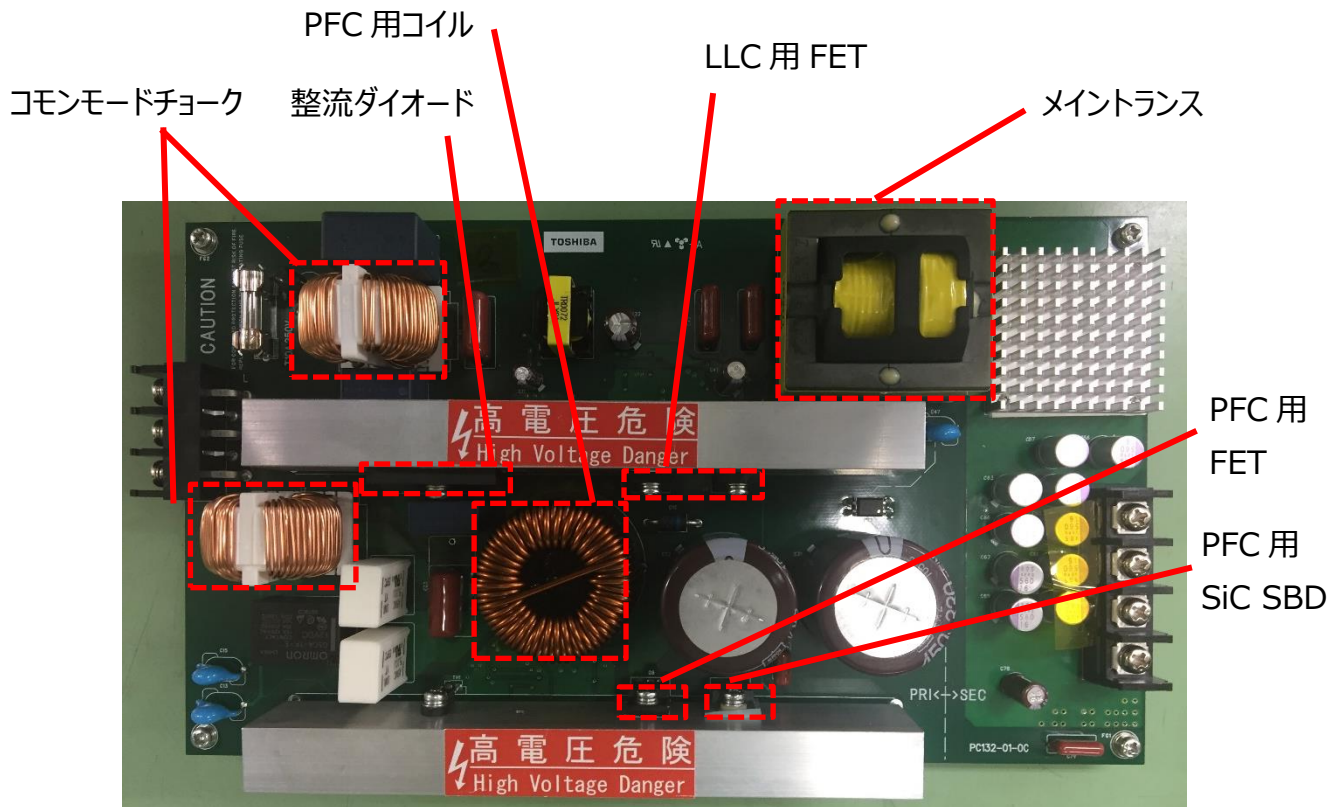
図 3.3 発熱量の大きな部品領域
