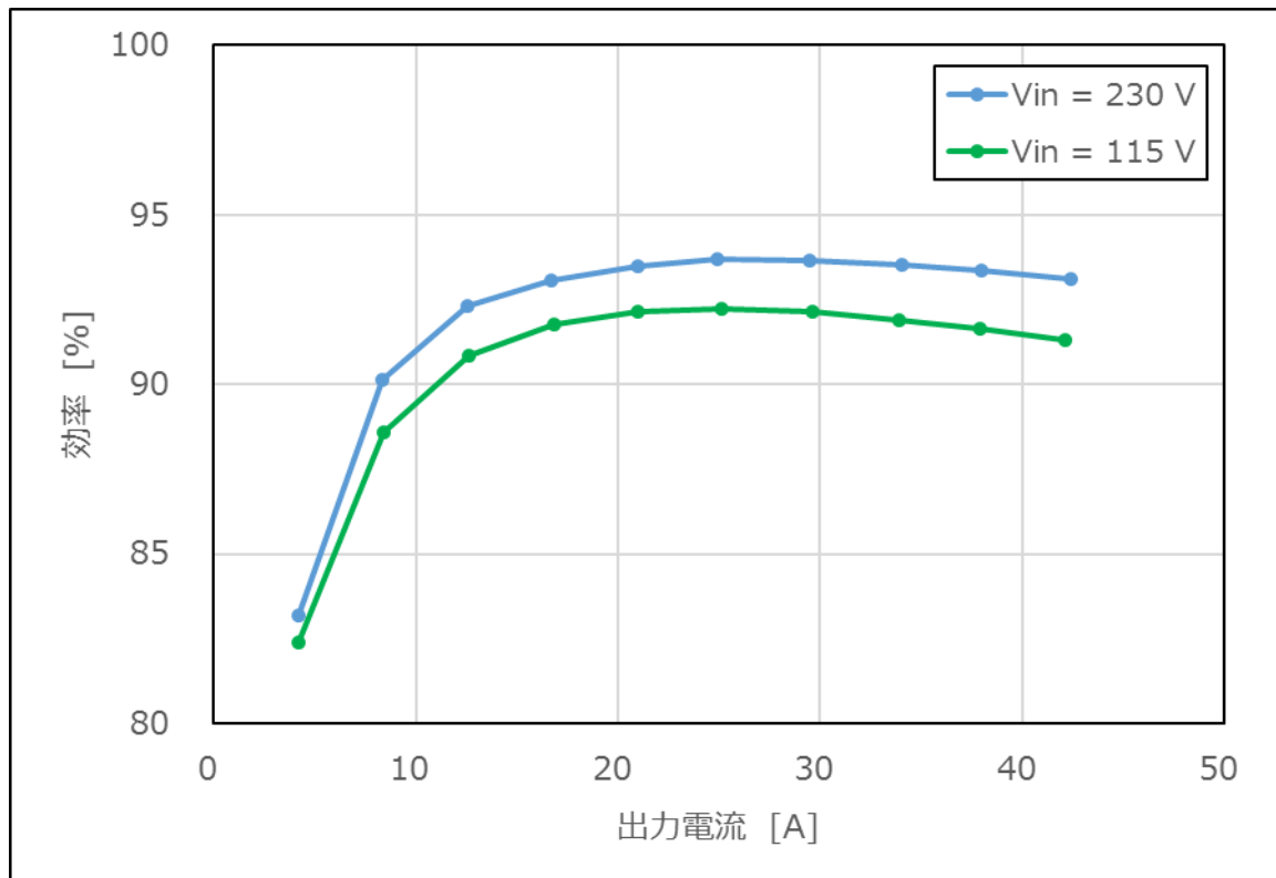
図 4.1 効率測定結果 (Vin = 115 V, Vin = 230 V)
