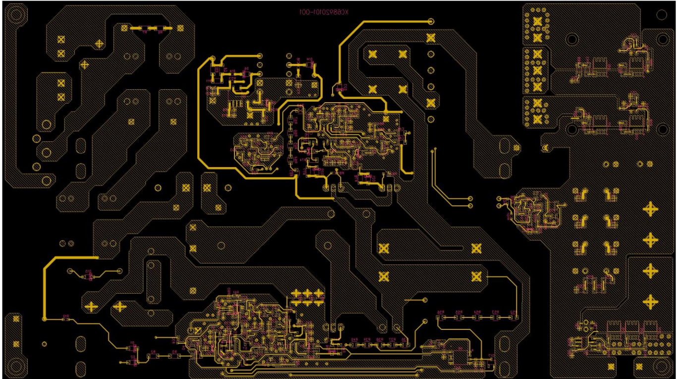
図 2.6 Layer2
