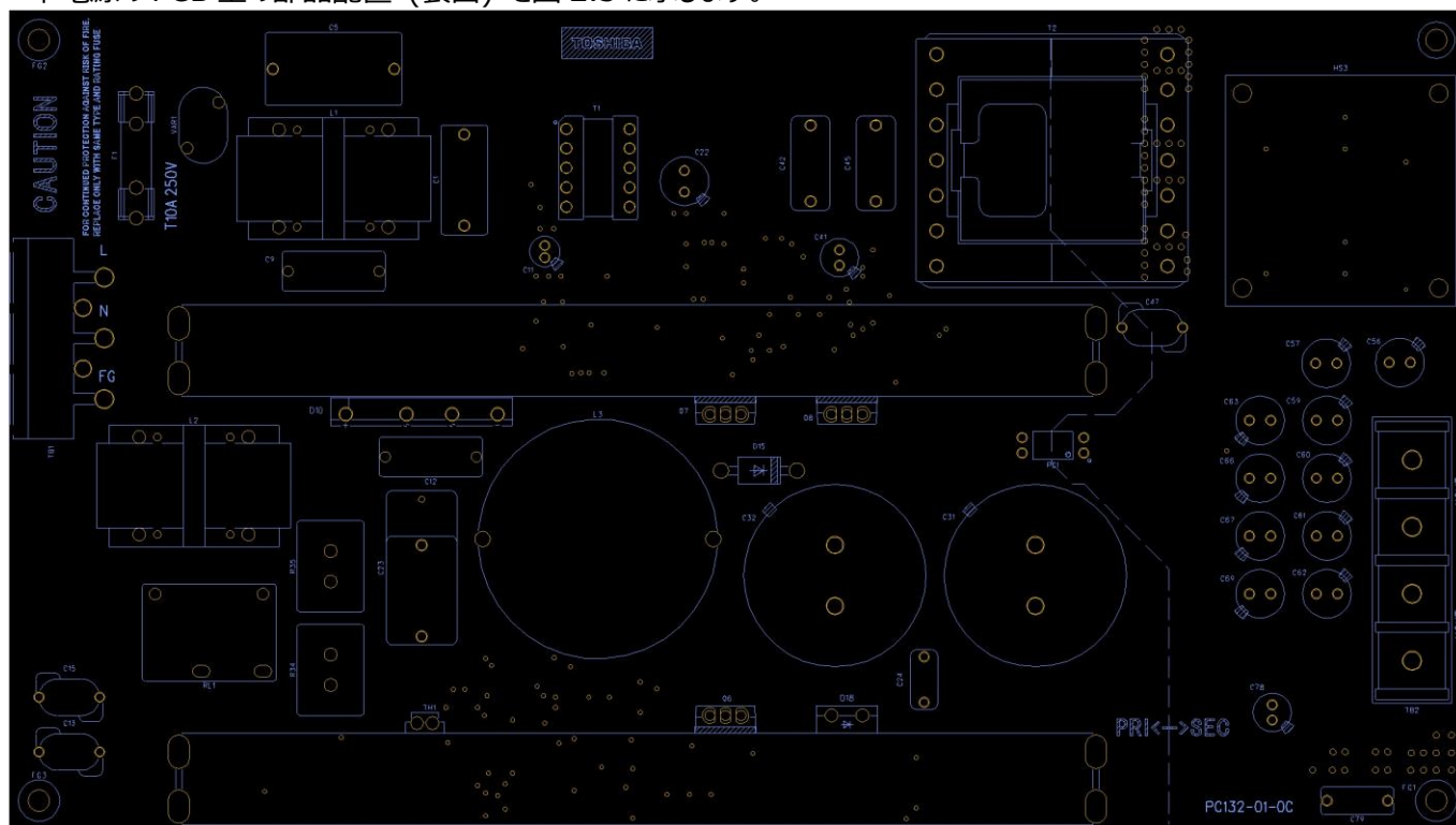
図 2.3 PCB 部品配置 (表面)
