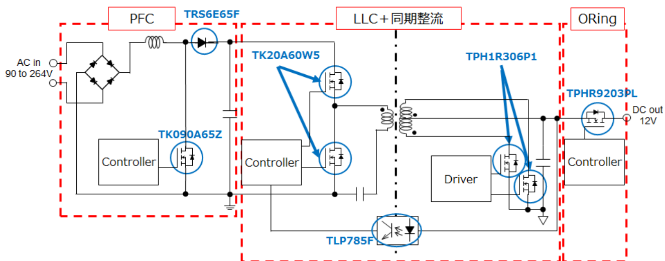
図 2.2 ブロック図
