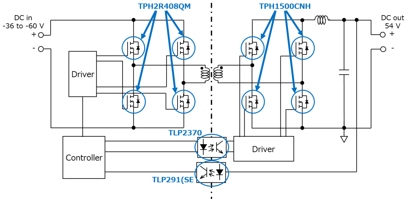
図 2.2 ブロック図
