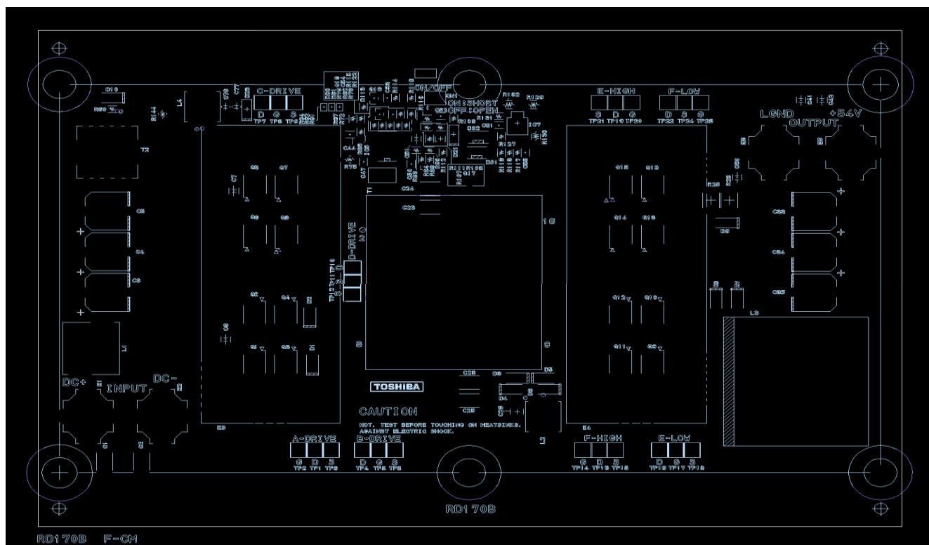
図 2.3 PCB 部品配置 (表面)
