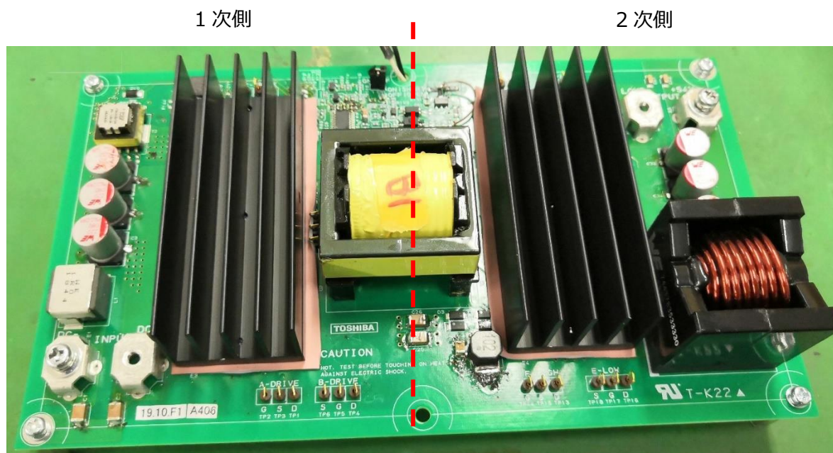
図 3.2 1次側領域と2次側領域
