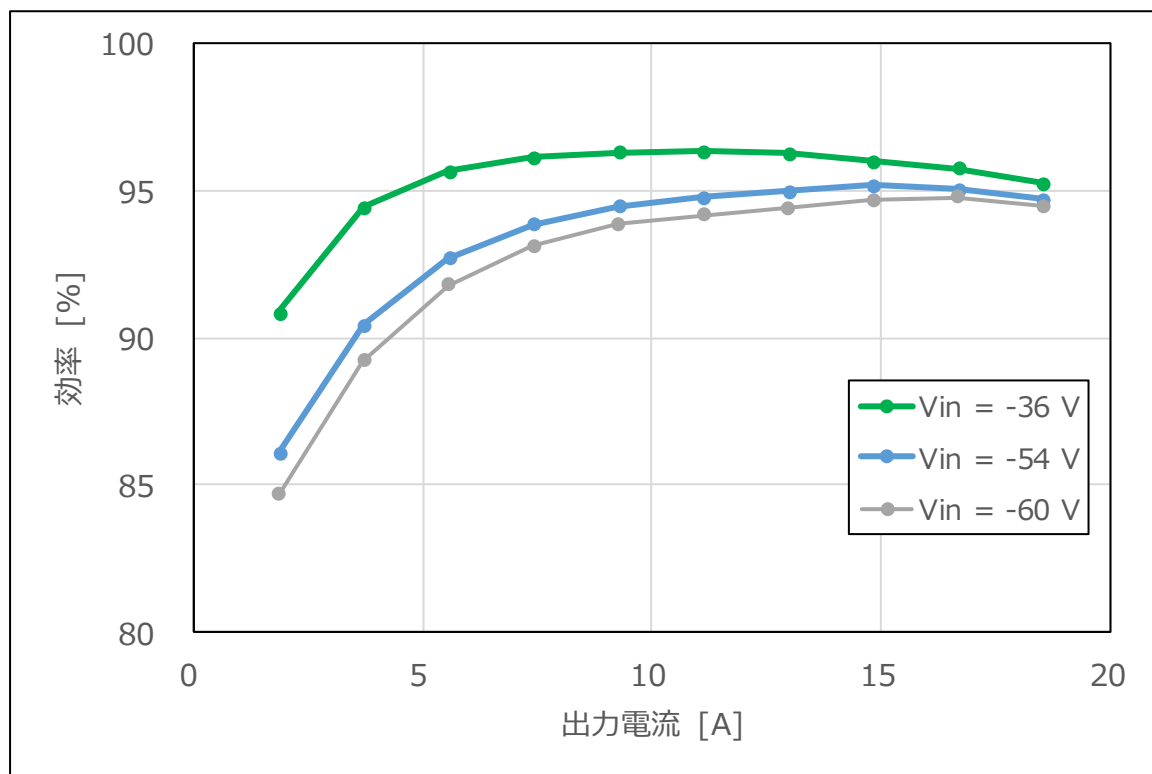
図 4.1 効率測定結果 ( V_{in} = -36\text{ V} , V_{in} = -54\text{ V} , V_{in} = -60\text{ V} )
