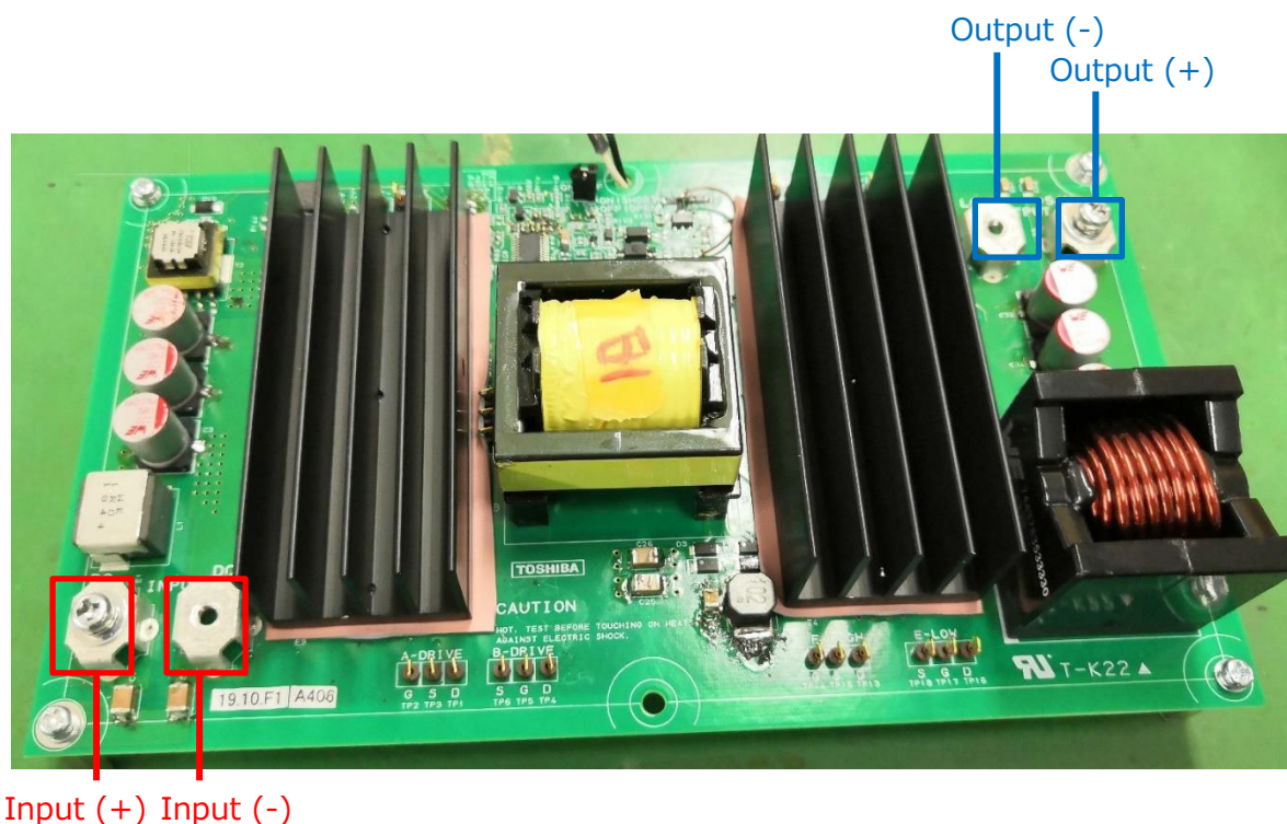
図 3.1 外部接続端子
