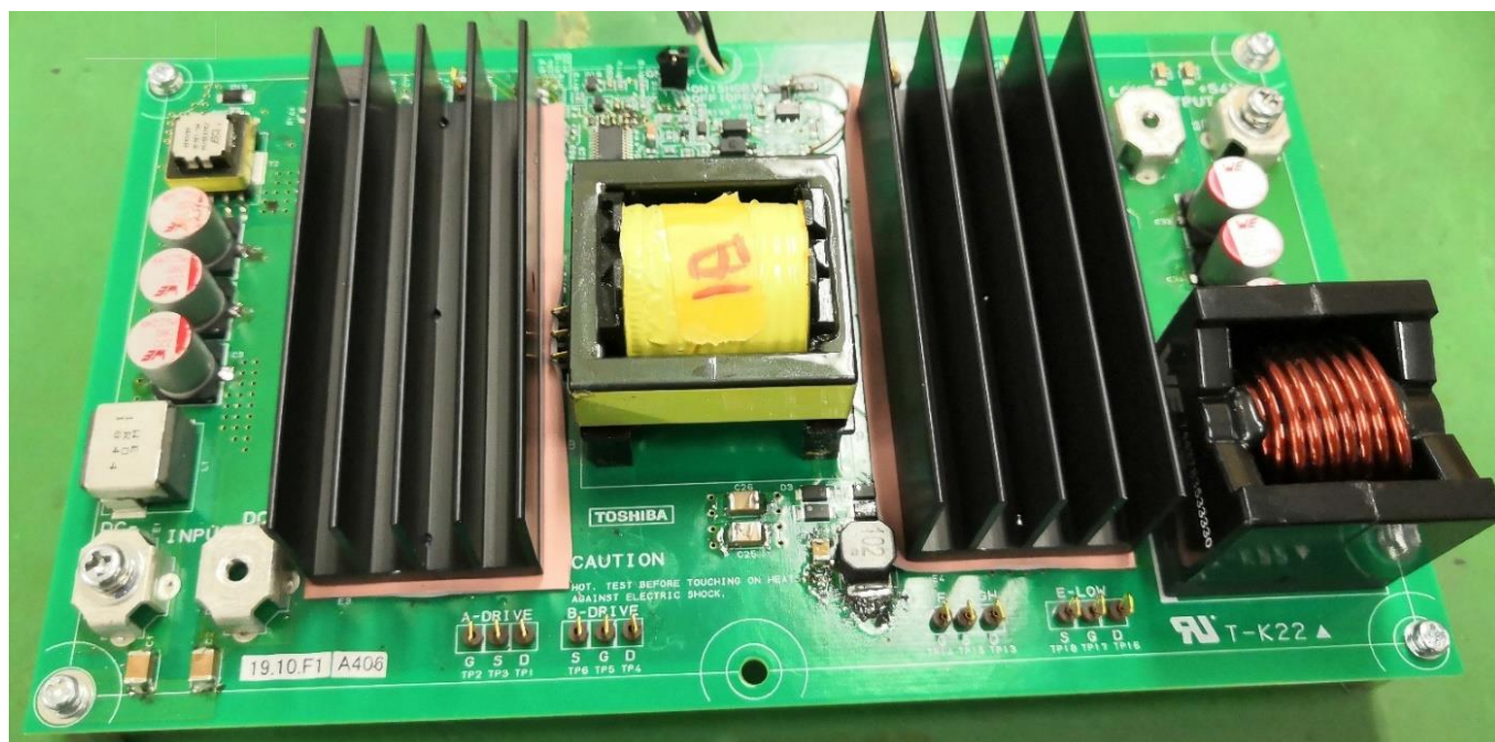
図 2.1 1 kW フルブリッジ方式 DC-DC コンバーター外観
