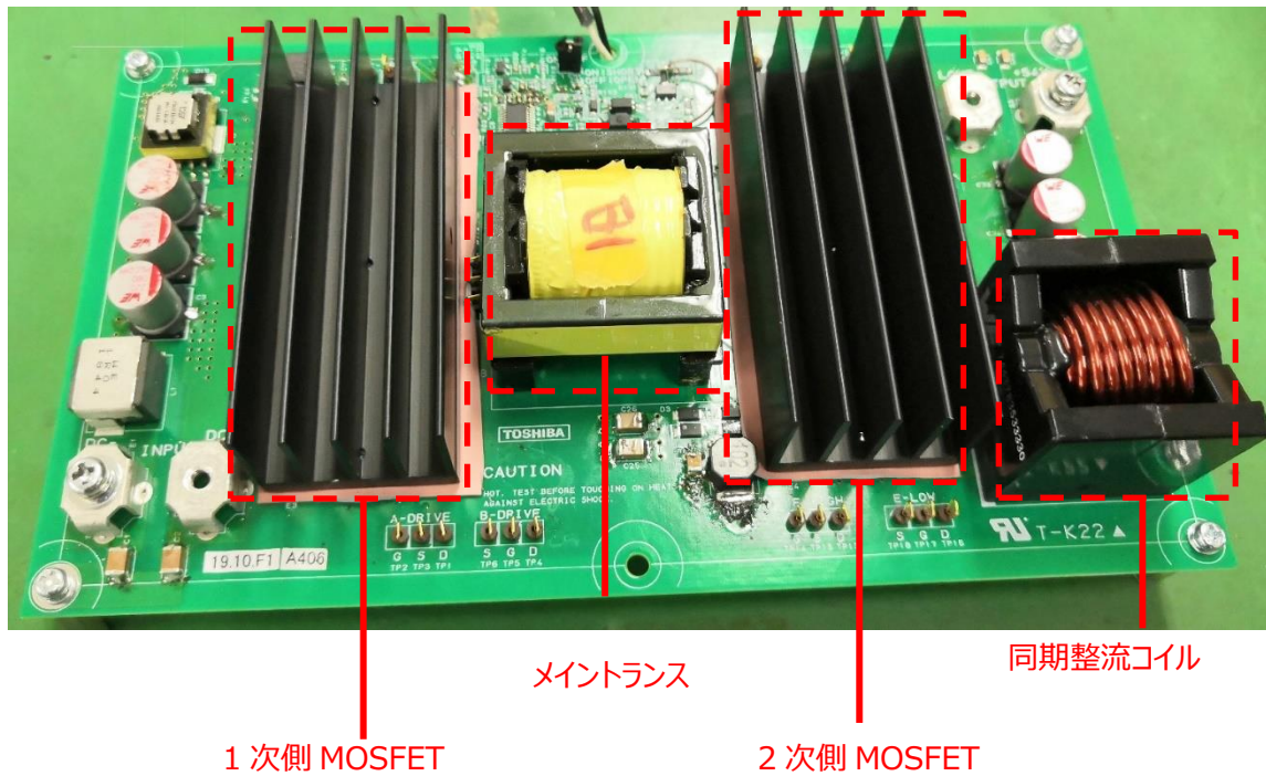
図 3.3 発熱量の大きな部品領域
