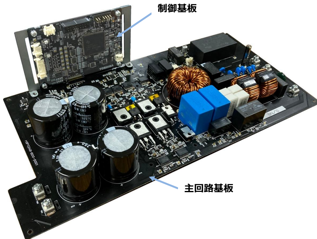
図 2.2 1.6 kW T 型 3 レベル方式 PFC 電源の側面写真
