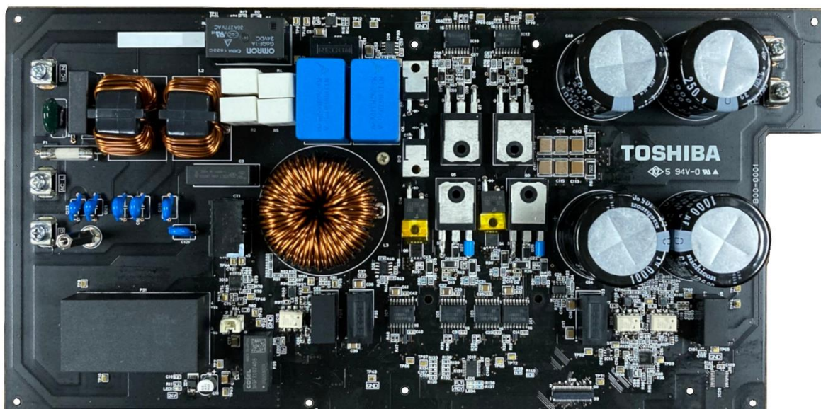
図 2.3 1.6 kW T 型 3 レベル方式 PFC 電源(主回路基板)の上面写真
