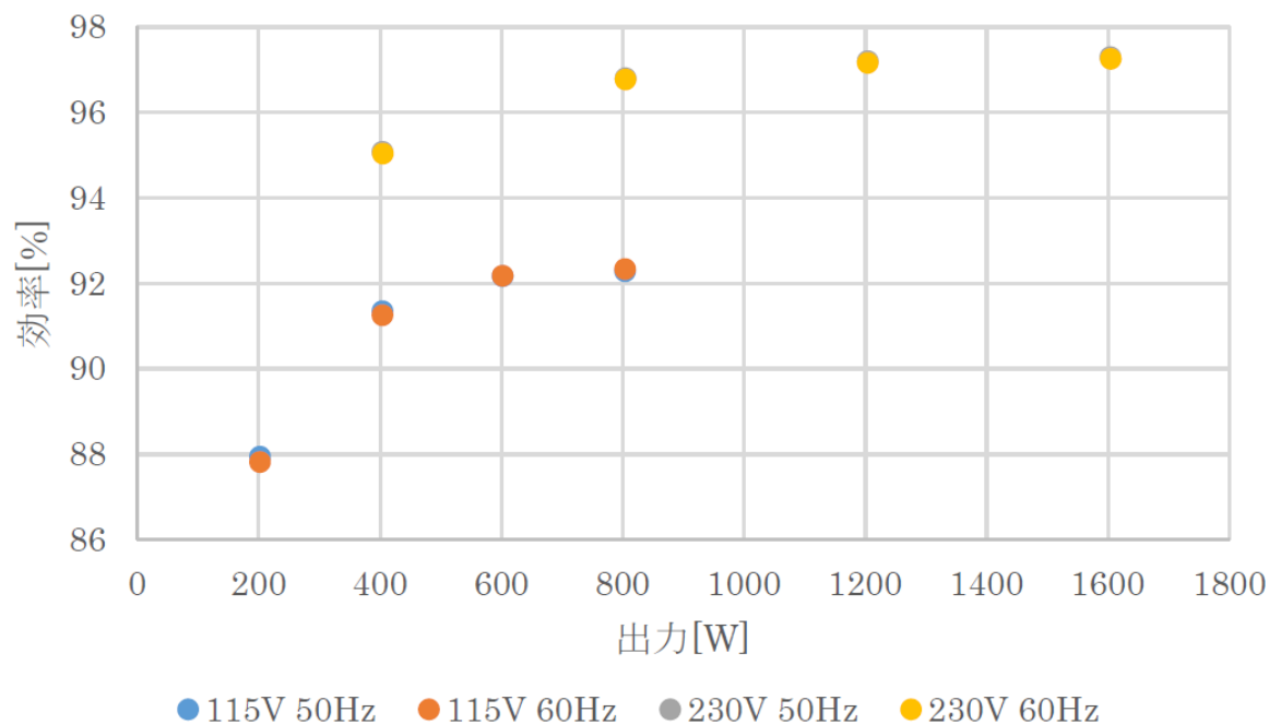
図 5.1 効率測定結果
