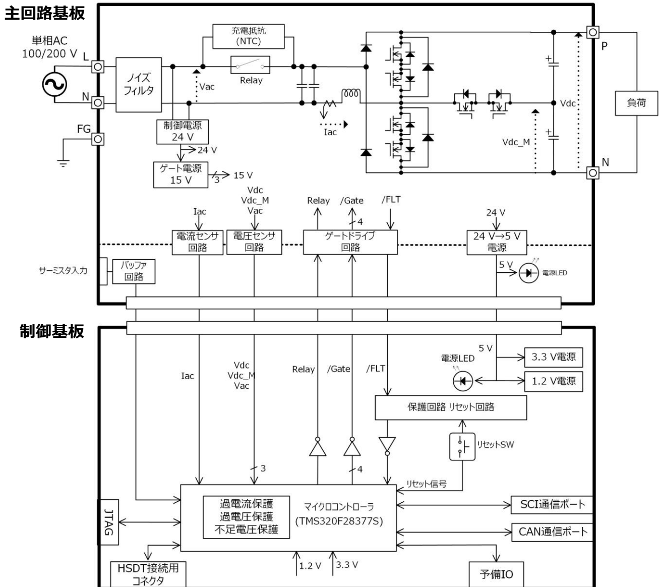
図 2.1 ブロック図
