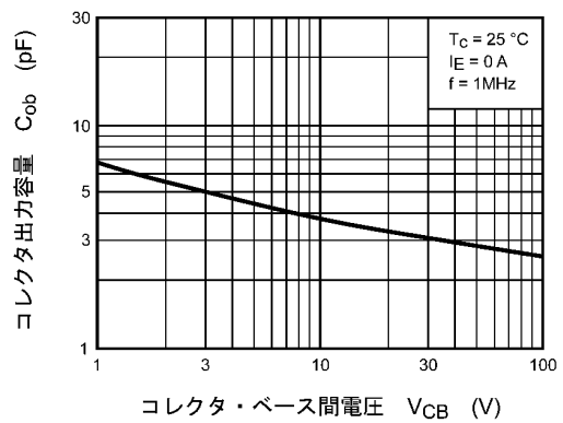
図 7.6 C_{ob} - V_{CB}
