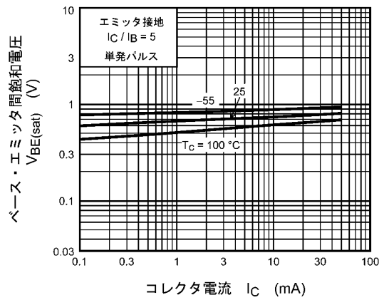
図 7.4 V_{BE(sat)} - I_C
