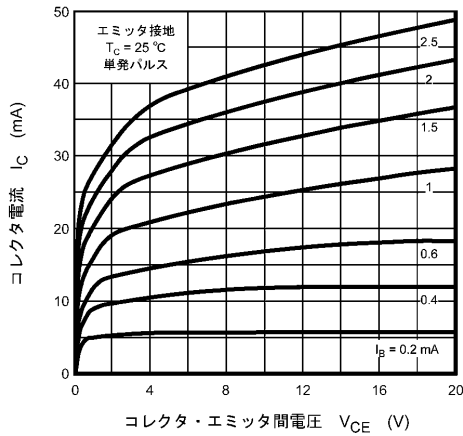
図 7.1 I_C - V_{CE}
