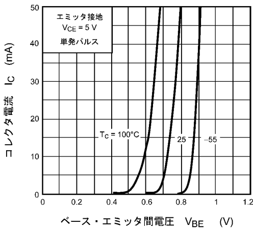
図 7.5 I_C - V_{BE}
