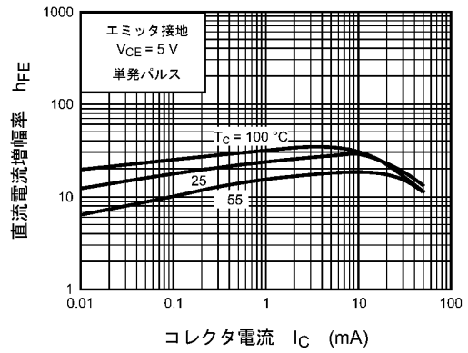
図 7.2 h_{FE} - I_C
