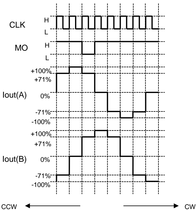
図 7.8.2 1-2 相励磁
