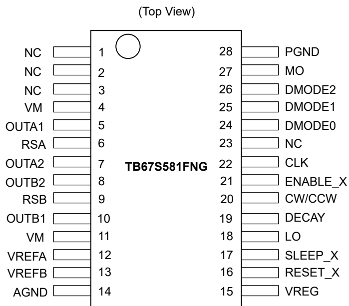
図3 ピン配置図
