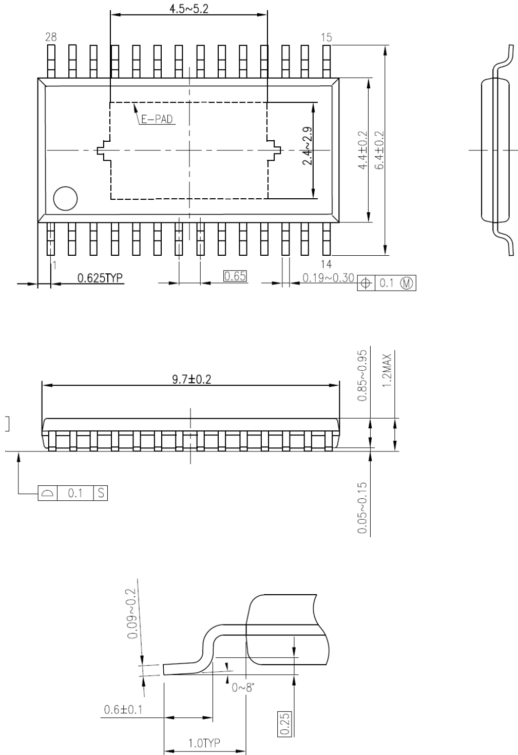
图 18 外形寸法图
