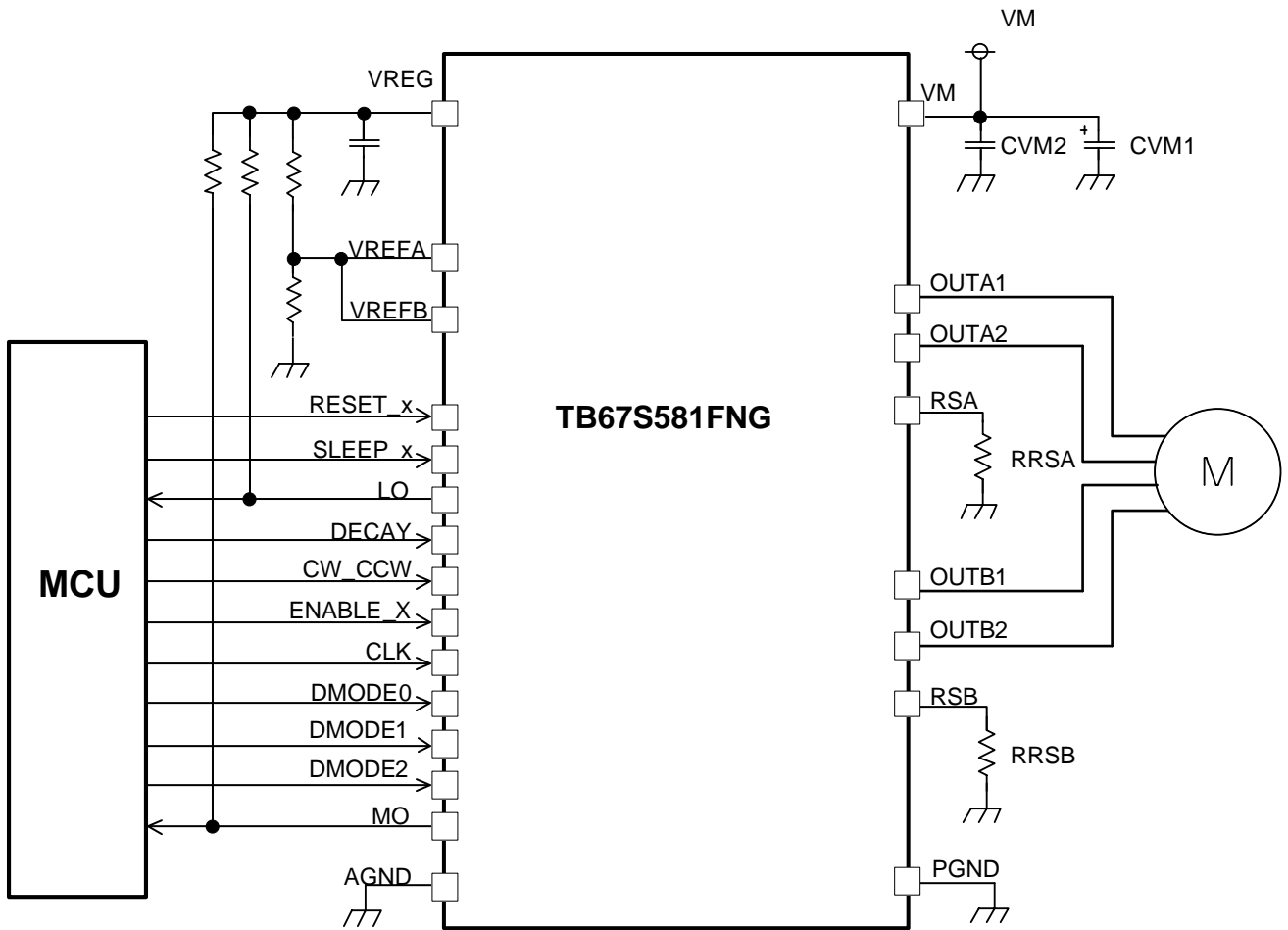
图 17 应用回路例
