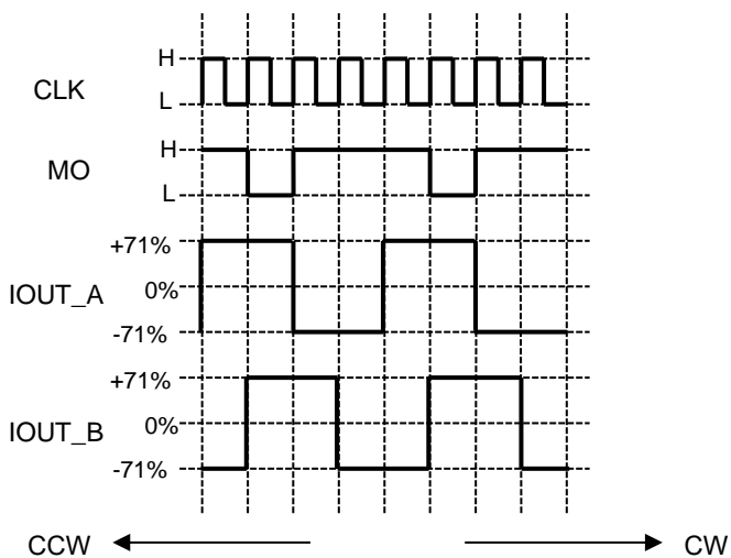
図 7.8.1 2 相励磁
