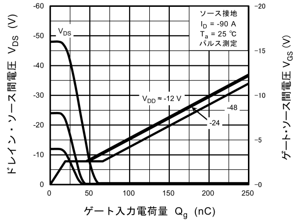
図 8.14 ダイナミック入出力特性
