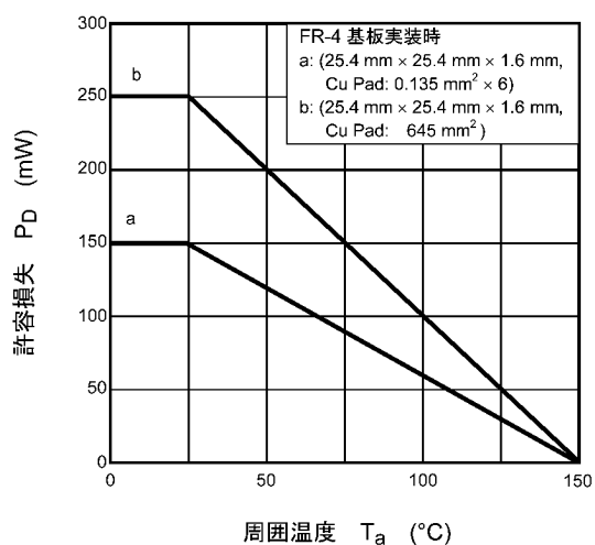
図 7.12 P_D - T_a
