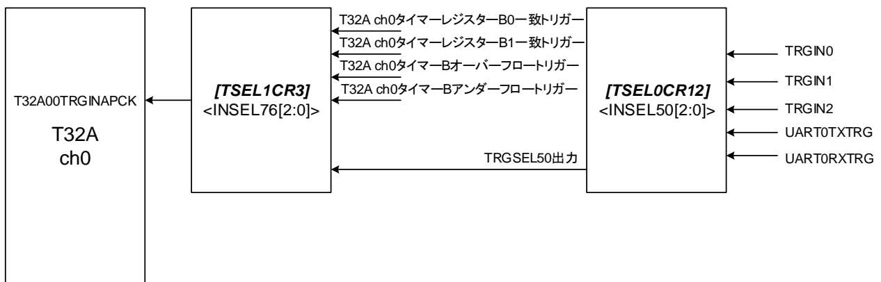
図 2.2 トリガーとTRGSEL接続概略図(T32A ch0)
