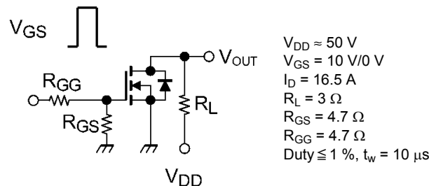
図 6.2.1 スwitching時間の測定回路例
