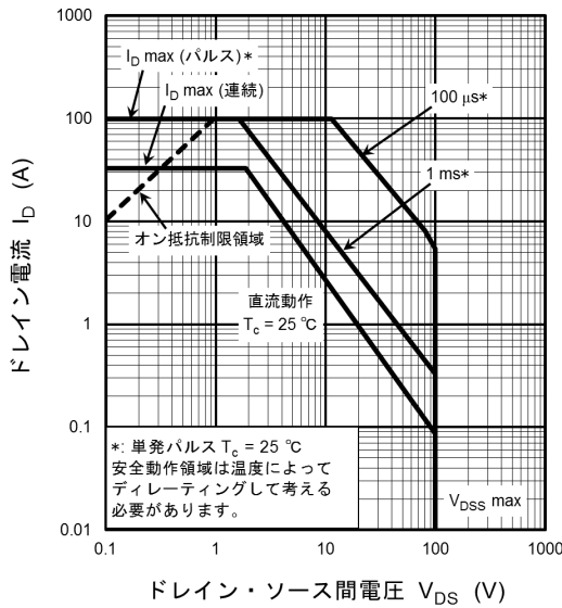
図 8.13 安全動作領域 (最大値 (保証値))
