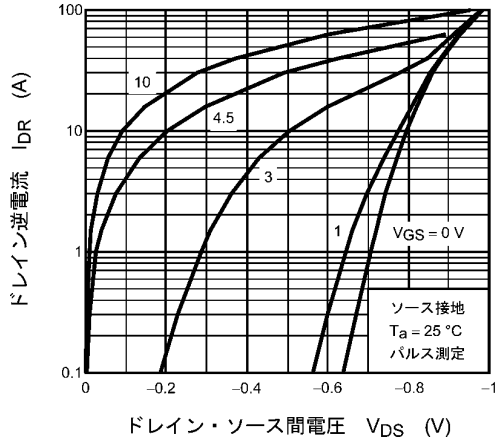
図 8.7 I_{DR} - V_{DS}
