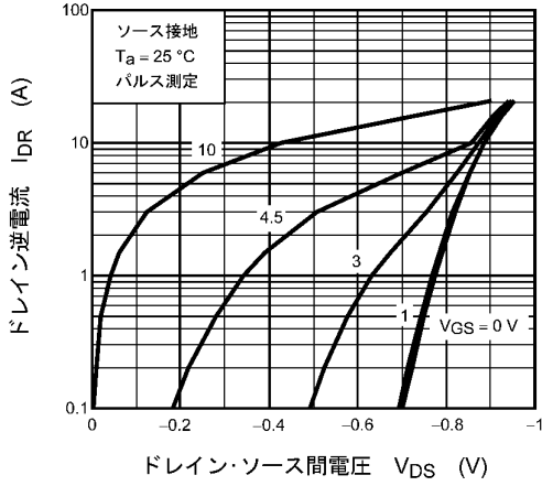
図 8.7 I_{DR} - V_{DS}
