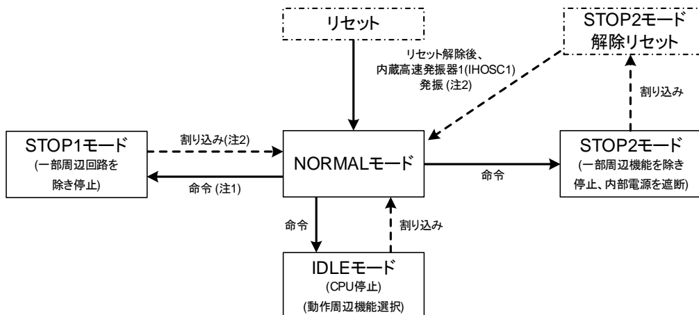
図 1.2 モード状態遷移
