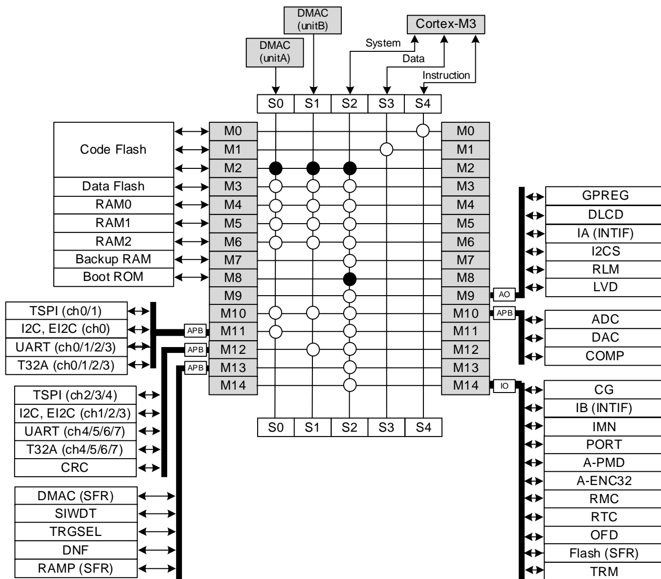
図 2.3 シングルチップモード
