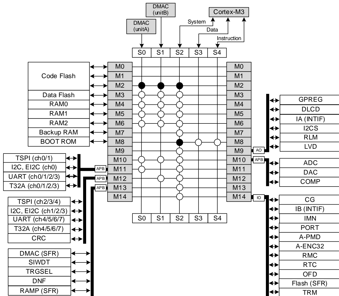
図 2.4 シングルブートモード
