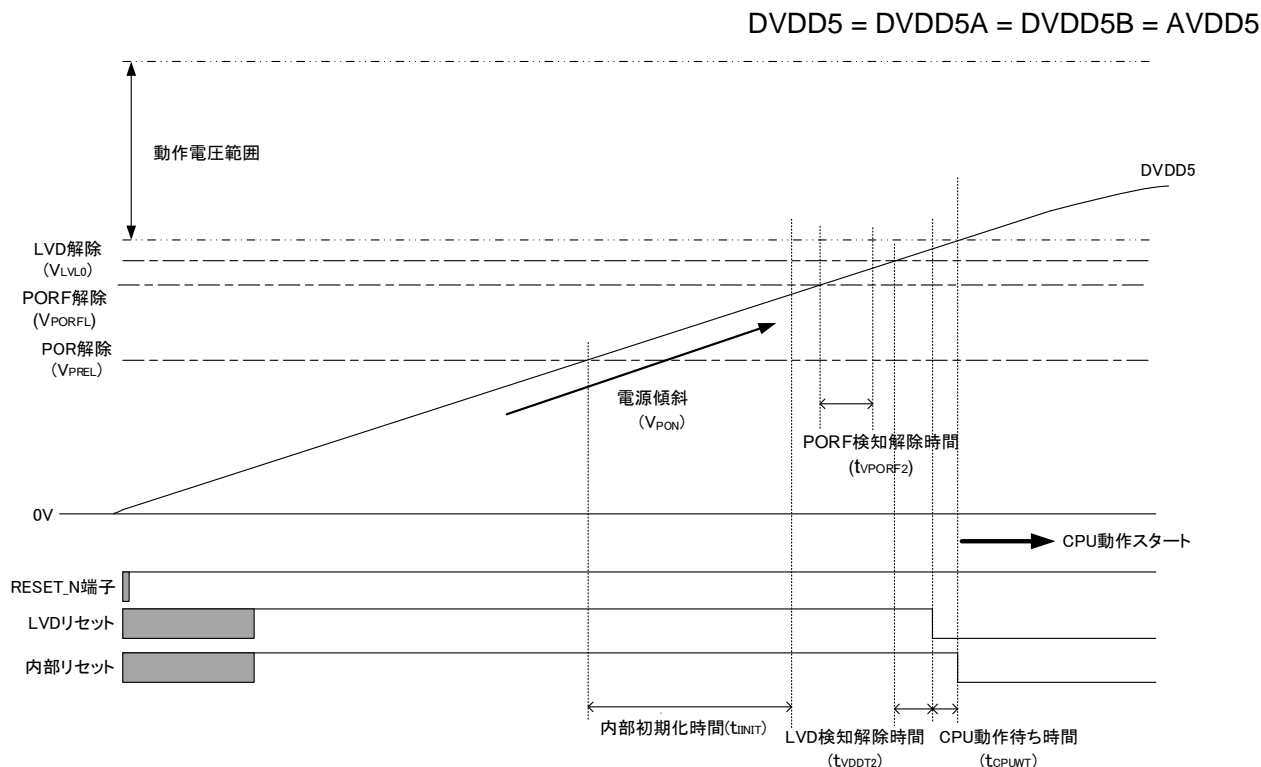
図 3.4 LVDリセットによるリセット動作
