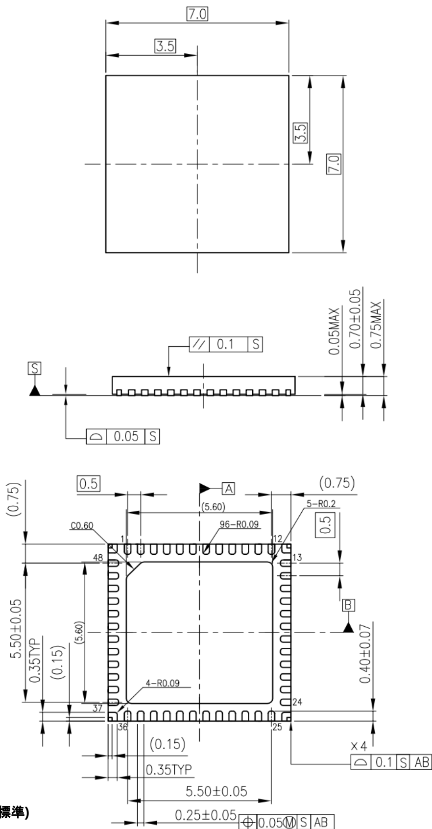
图 11.1 外形寸法图
