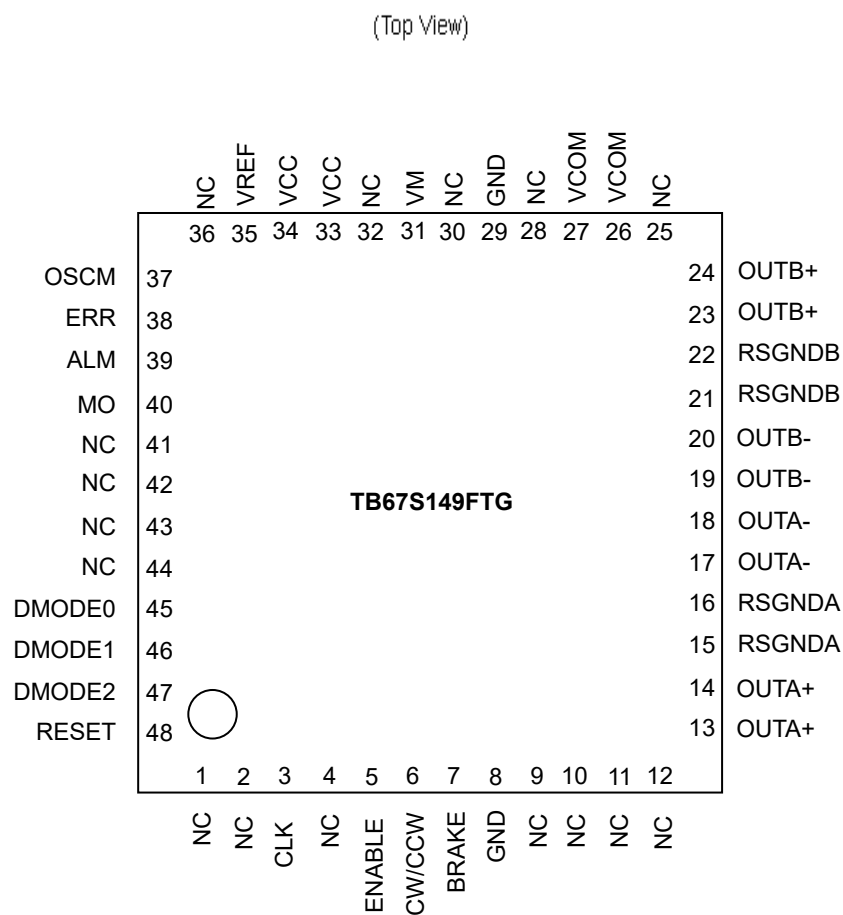
図 4.1 端子配置図
