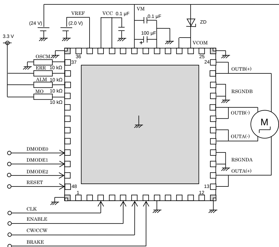
図 10.1 応用回路例
