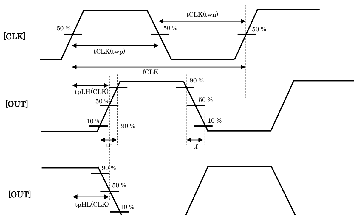
図 9.1 AC 特性タイミングチャート
