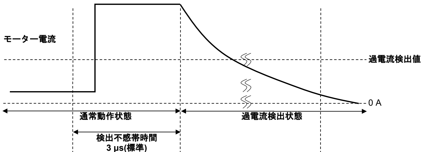
図 6.7 過電流検出タイミングチャート
