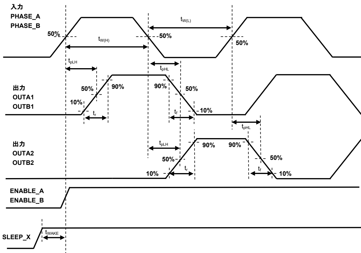
図 9.1 AC 特性タイミングチャート
