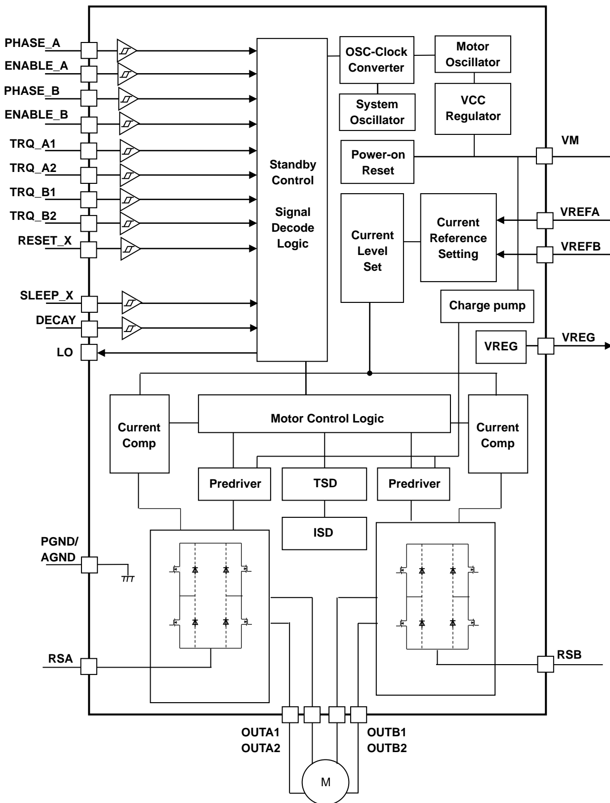
図4 ブロック図
