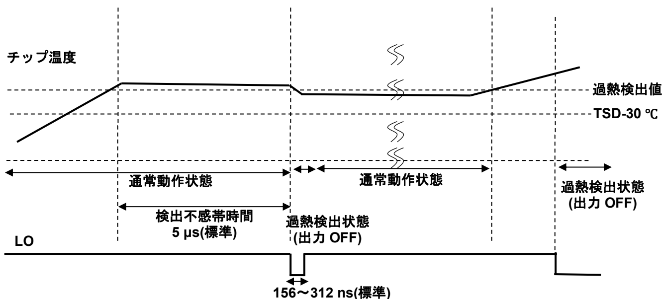
図 6.6 過熱検出のタイミングチャート 2
