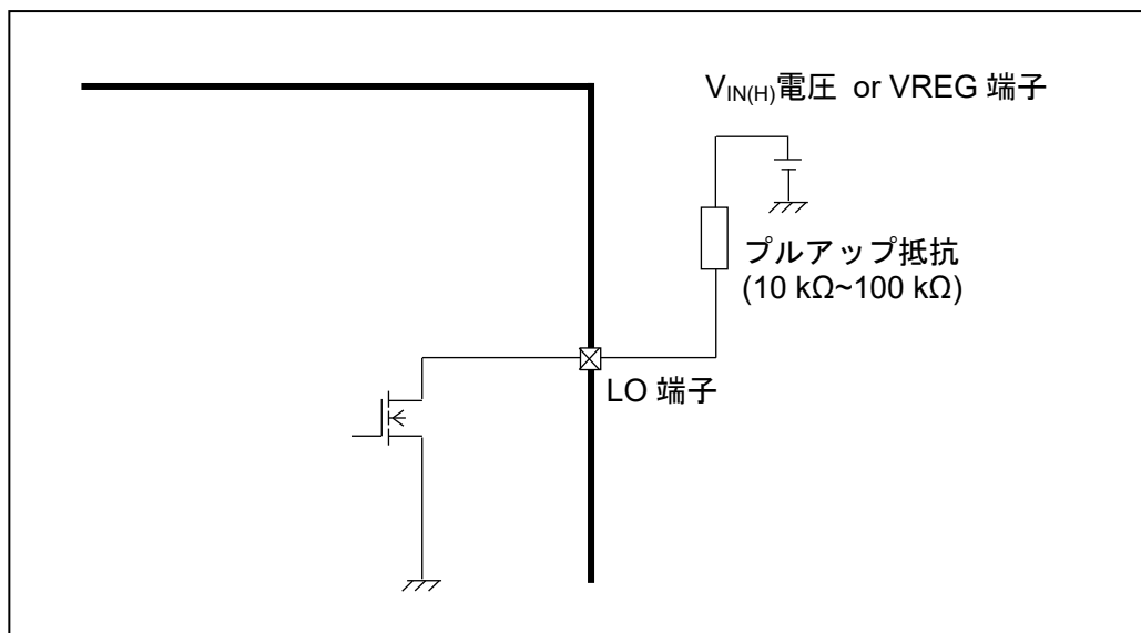
図 6.1 LO 端子等価回路図
