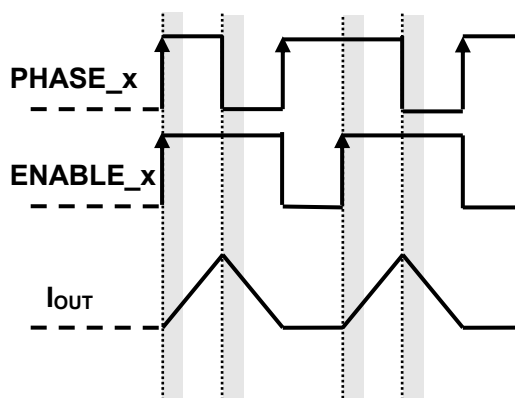
図 6.3 入力信号と t BLK の不感帯時間タイミングチャート
