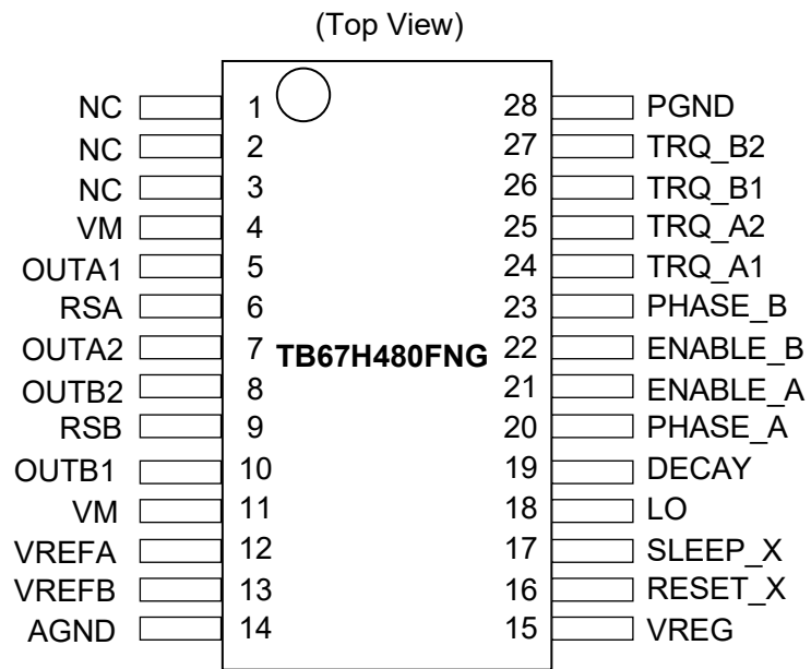
図 3.1 ピン配置図
