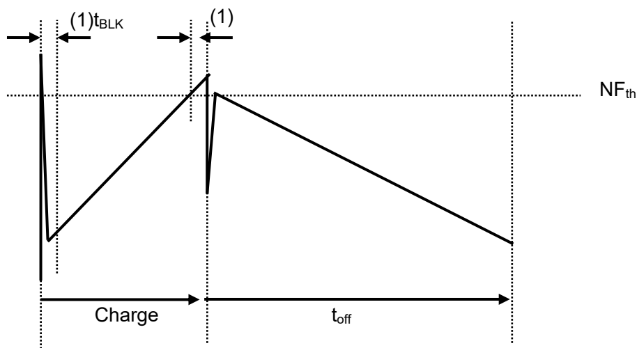
図 6.2 定電流 PWM タイミングチャート
