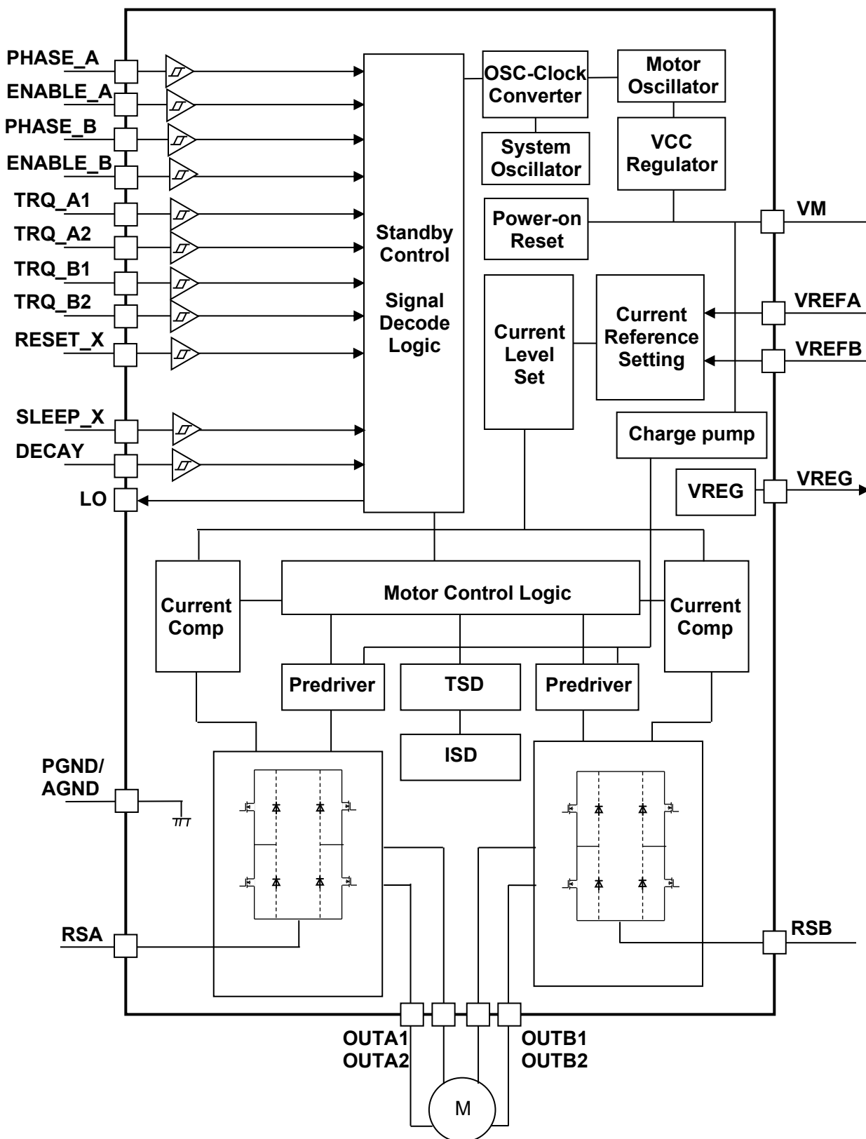
図 4.1 ブロック図
