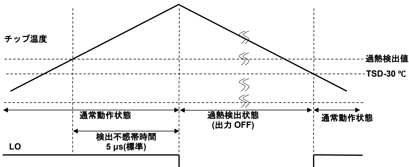
図 6.5 過熱検出のタイミングチャート 1
