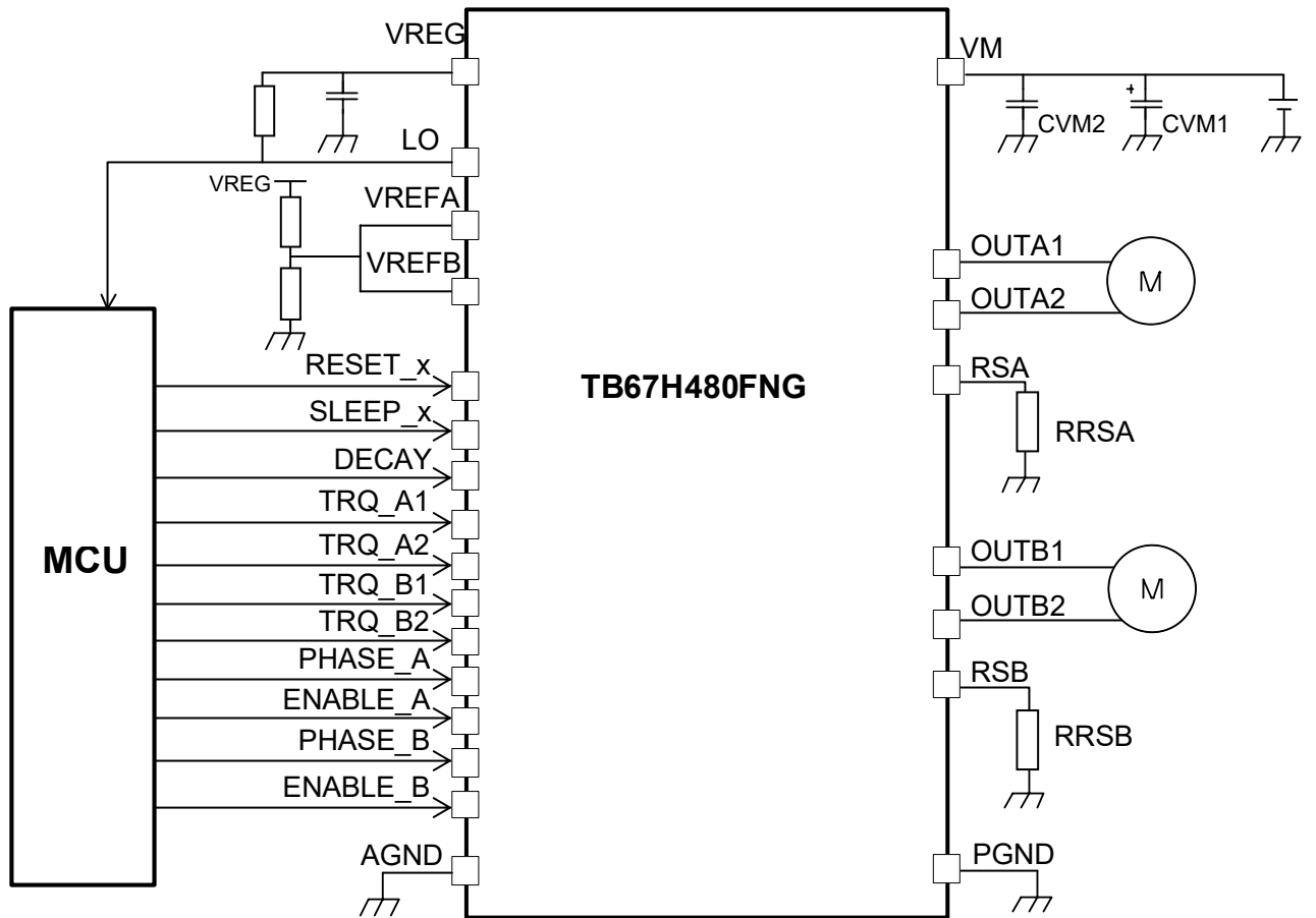
图 10.1 応用回路例
