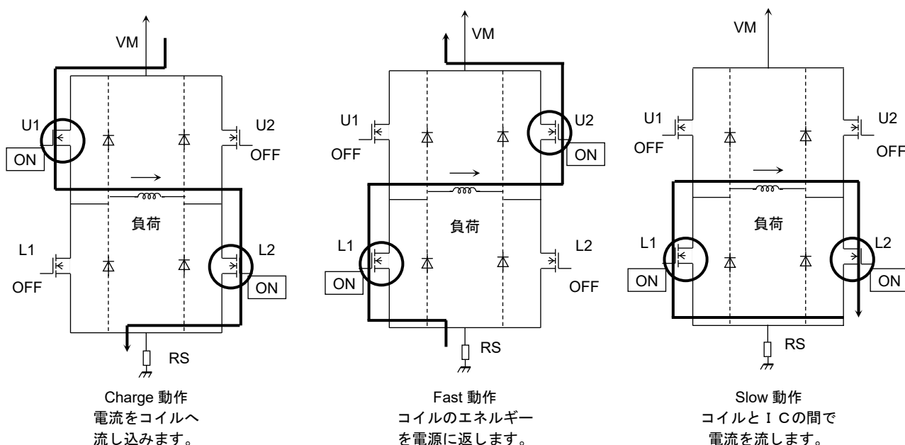
図 6.4 出力トランジスタ動作モード
