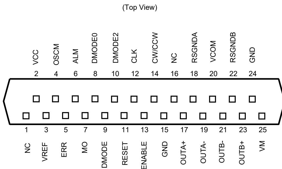
图 4.1 端子配置图
