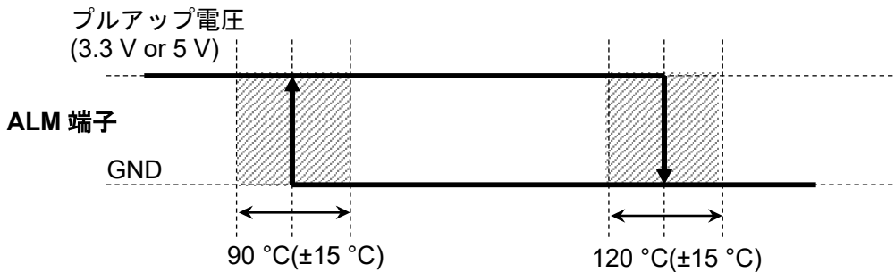
図 6.3 ALM 端子設定
