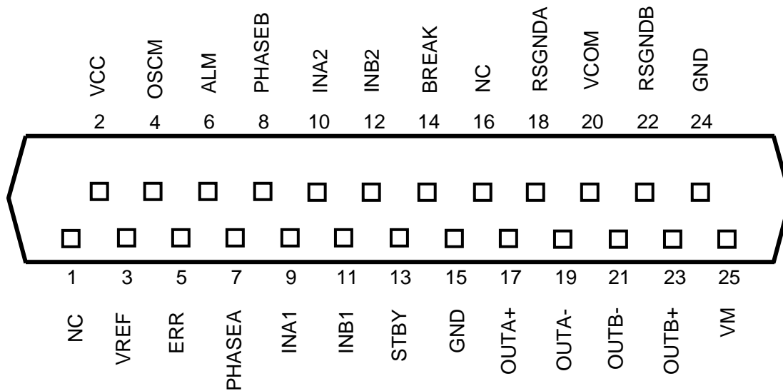
图 4.1 端子配置图
