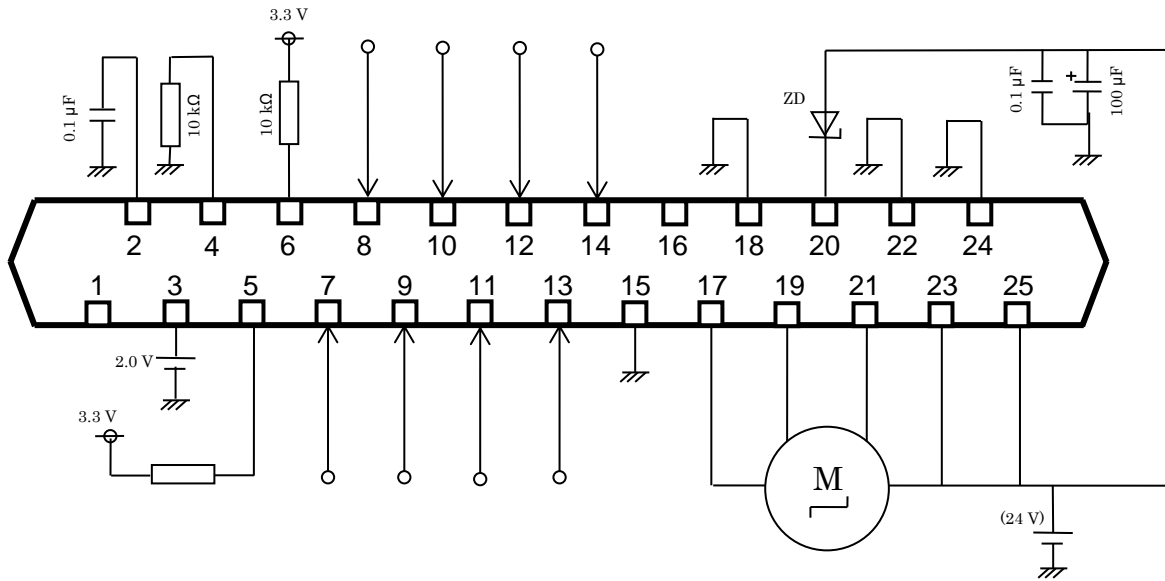
図 10.1 応用回路例
