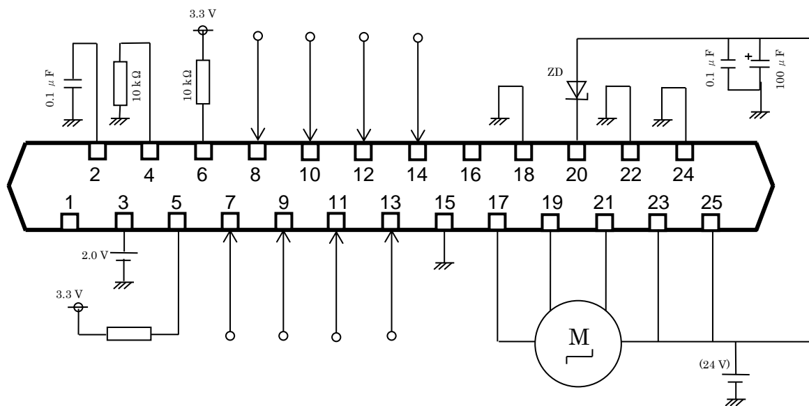
図 10.1 応用回路例
