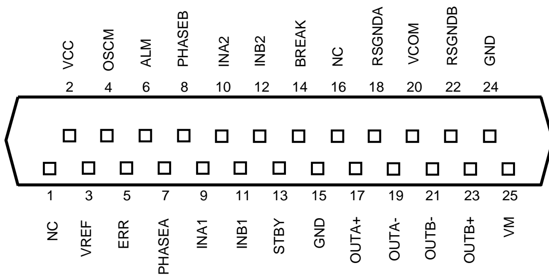
图 4.1 端子配置图
