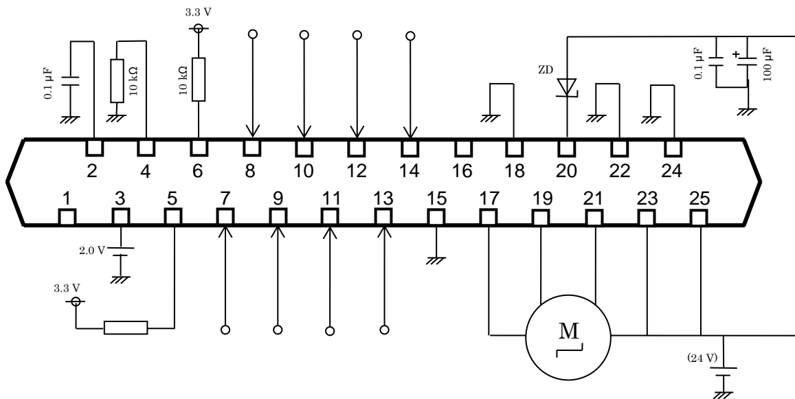
図 10.1 応用回路例
