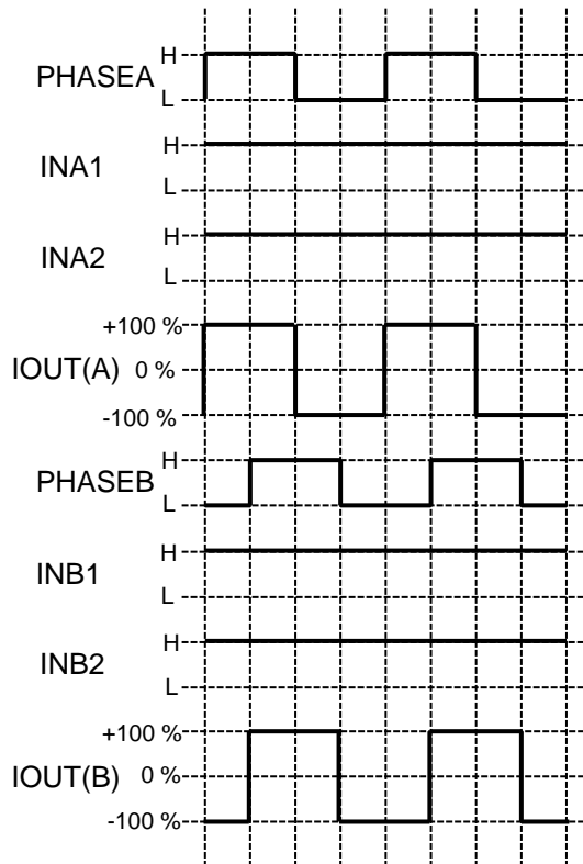
図 6.2 2 相励磁のタイミングチャート
