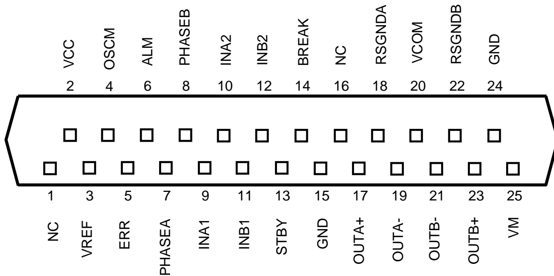
图 4.1 端子配置图
