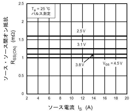
図 9.2 R_{SS(ON)} - I_S
