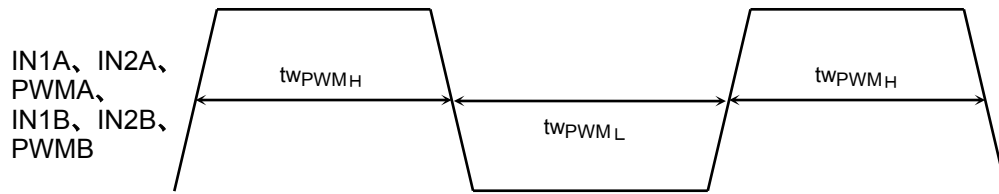
图 1 波形と名称
