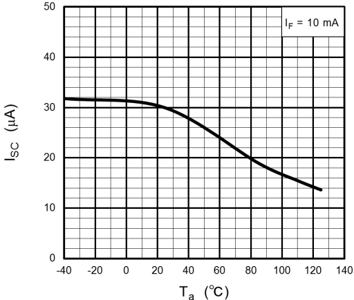
Fig. 12.7 Isc - Ta
