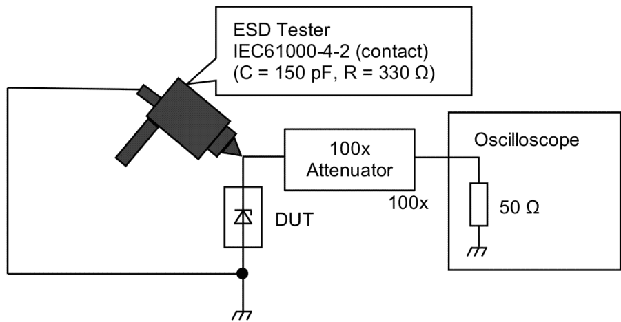
Fig. 9.3 IEC61000-4-2 (Contact)
